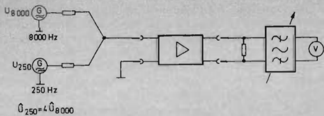
Fig 13 Mätuppkoppling för bestämning av internmodulationsdistorionen.
