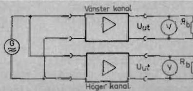
Fig 14 Mätuppkoppling för kontroll av kanallikheten hos en stereoförstärkare.
