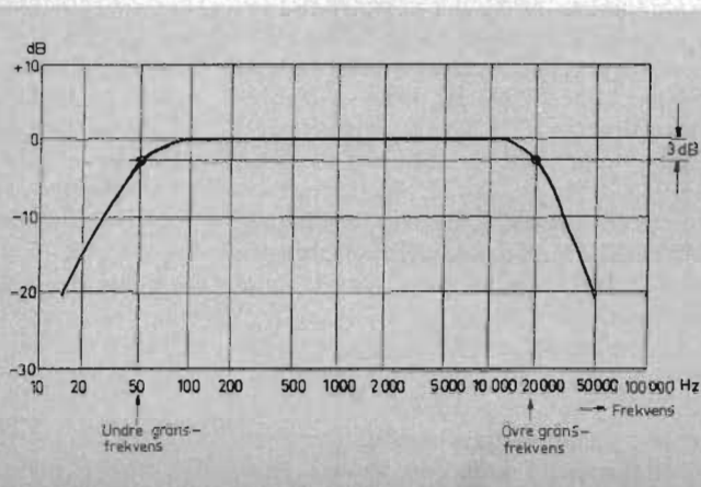
Fig 7 Kurvor av detta slag visar en förstärkares frekvensgång och frekvensområde, det senare anges oftast som den frekvensbana inom vilken förstärkarens utspänning inte sjunker mer än 3 dB.
