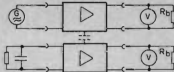
Fig 15 Mätuppkoppling för kontroll av överhörningsdämpningen i en stereoförstärkare. Den streckade kondensator som antyds mellan de båda förstärkarkanalerna symboliserar »läckningen» mellan kanalerna.
