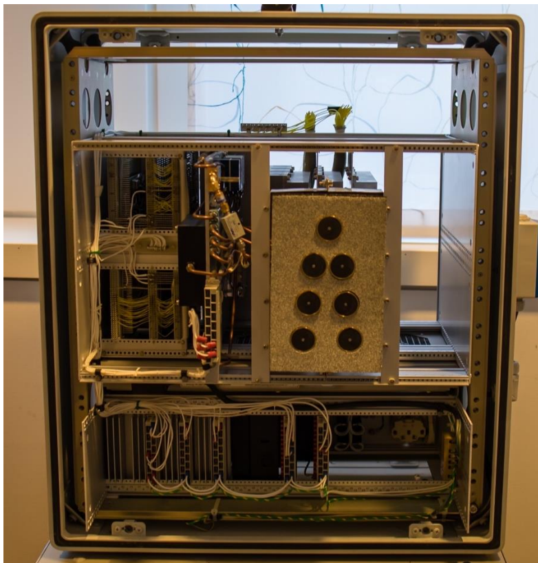
Interferometer, försöksutrustning
