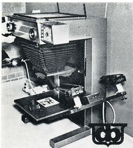
Reproduktionskamera GRAFEX automatic.
