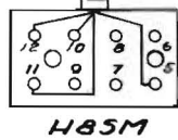
Ledningsplan (ritning FR-3748)
