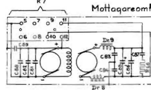
Mottagareomformare
