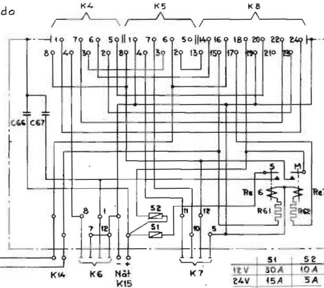
Mottagareomformare
