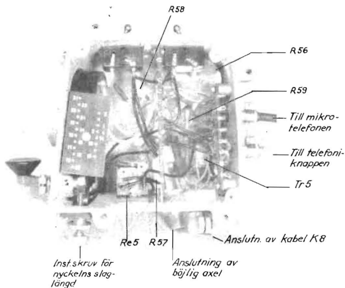
Fig 16. Betjäningsapparaten
