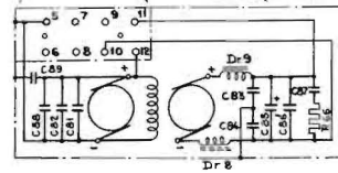
Mottagareomformare
