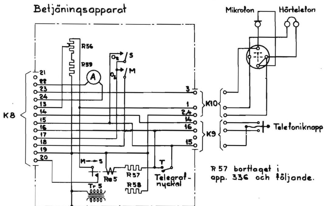
Fig 17. Kopplingschema för betjäningsapparaten.
