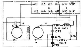
Sändareomformare
