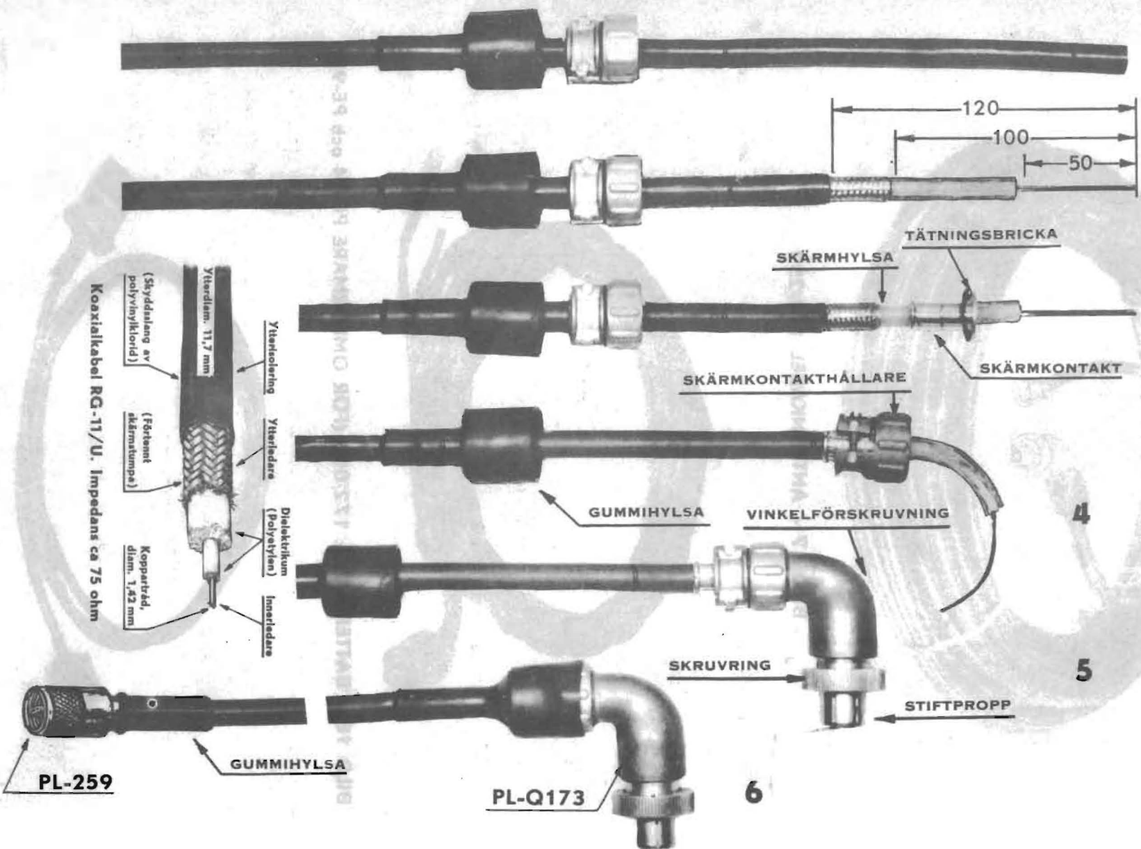
BILD 20 - KOPPLINGSANVISNING FÖR ANTENNKABEL 173/259
