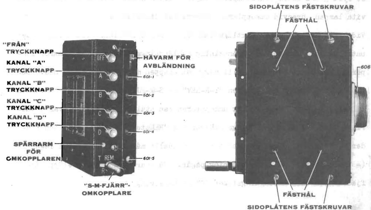
BILD 4 - MANÖVERAPPARAT BC-602-B
