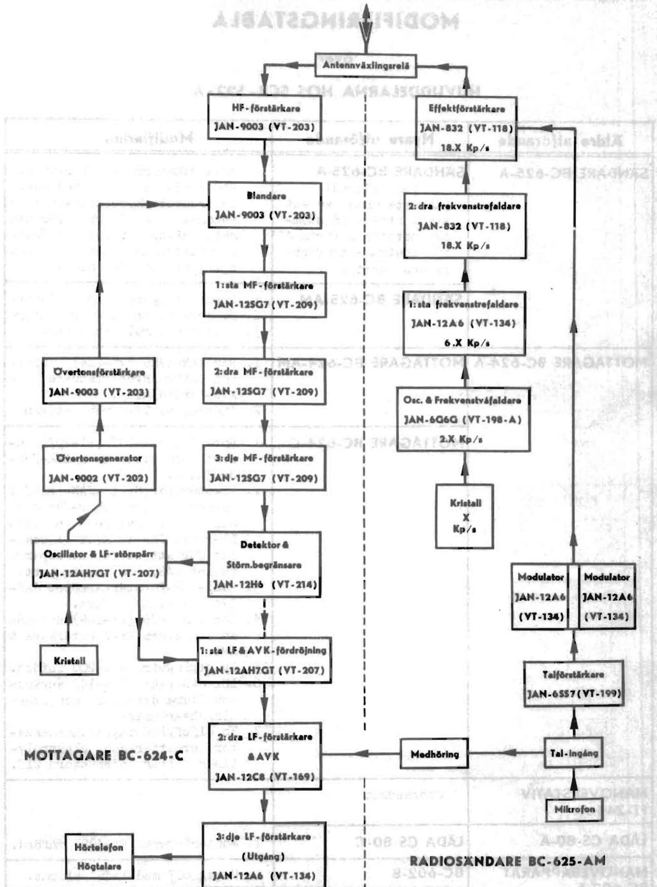
BILD 24 – BLOCKSCHEMA ÖVER MOTTAGARE BC-624-C OCH SÄNDARE BC-625-AM
