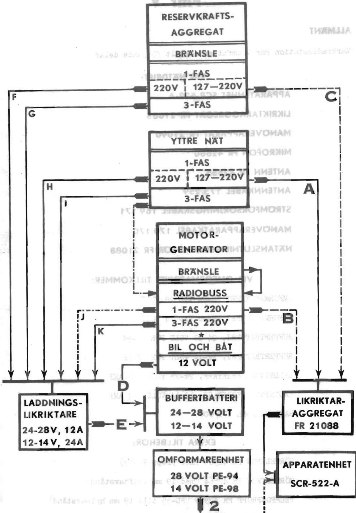
BILD 6 - STROMFORSÖRJNINGSSCHEMA FOR Fmr V
