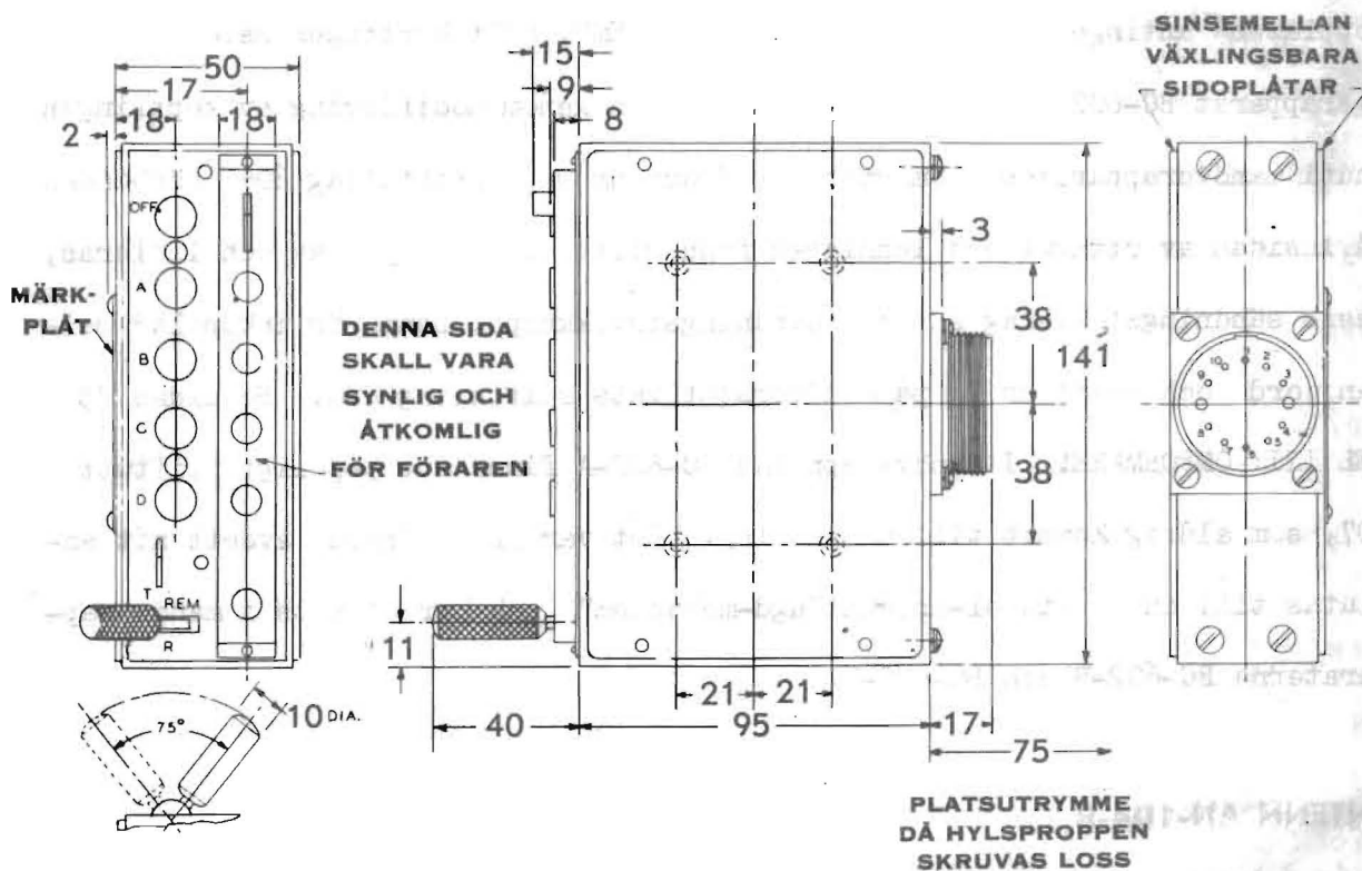
BILD 4 - MANÖVERAPPARAT BC-602-B
