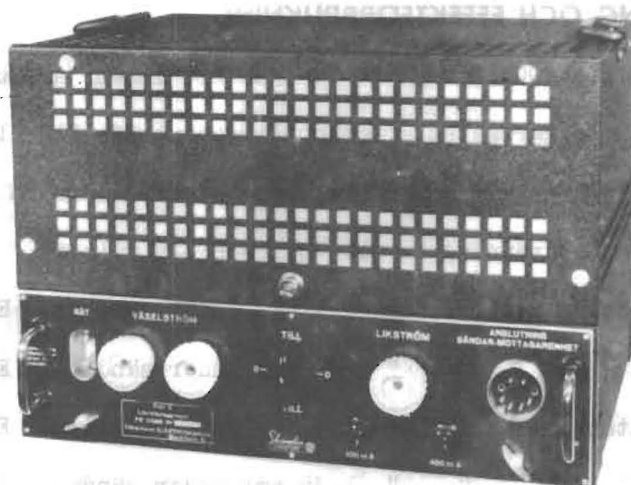
BILD 7 - LIKRIKTARAGGREGAT FR 21088 SETT FRAMIFRÅN
