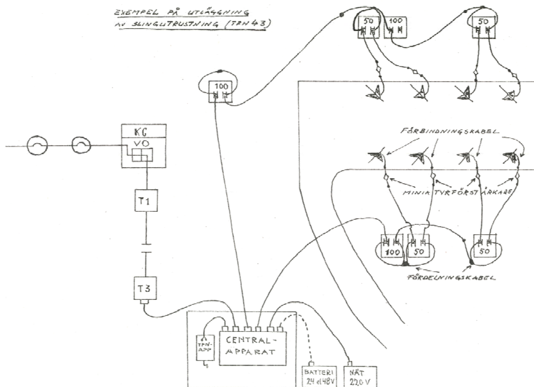
Slingutrustning Tfn 43.
