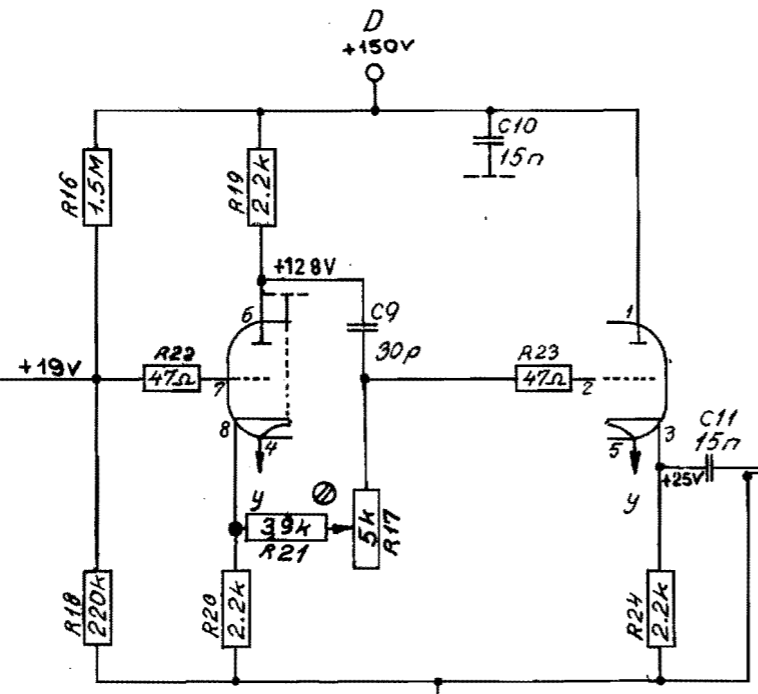
V3 E188CC Phase shifter
