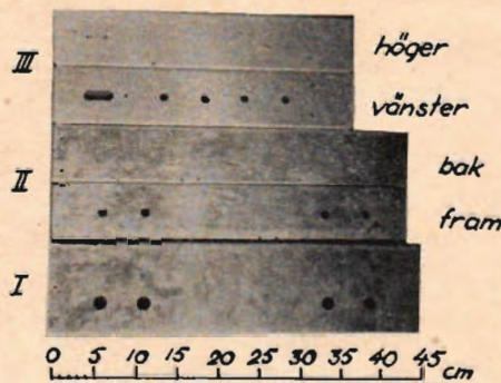
Fig. 1 (t. v.): Yttermåttarna på ramens delar. I är stöd för bildröret. II är gavlar. III är fram- och bakstycke, varav framstycket ska vara något kortare för att passa mellan gavlarna. Fig. 2 (nedan): Ramens delar med borrade hål. Fig. 3 (t. h.): Den färdigmonterade ramen.
