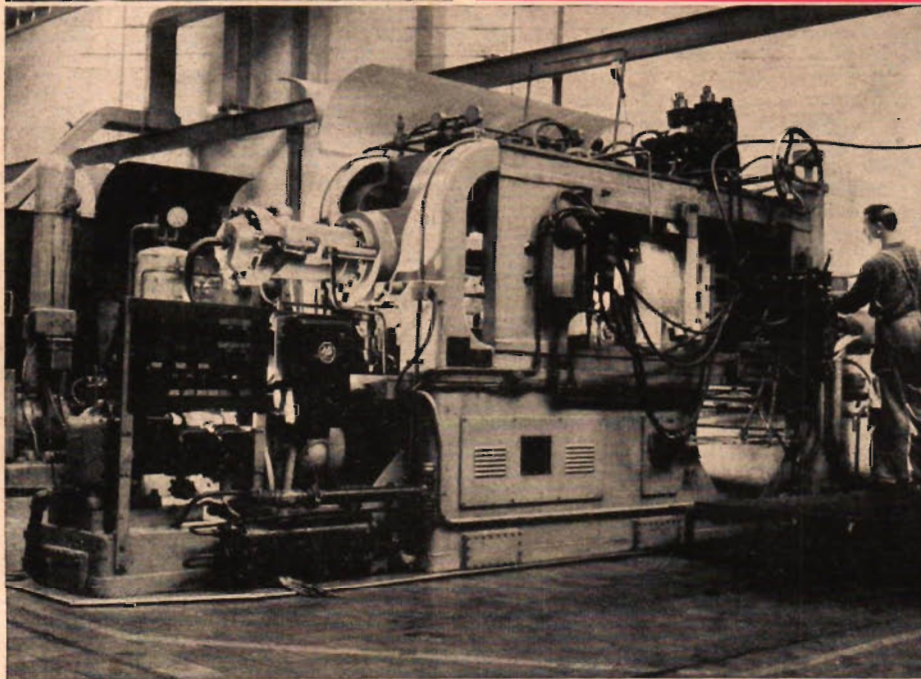
F. v.: Pressgjutningsmaskin, fabriken Cleveland, typ kalkkammare. Nedan: Detta är den största seriebyggda pressgjutningsmaskin som tillverkats — det finns bara en i Sverige. På översidan syns en påmonterad anordning för dragning av slider. Maskinen, fabriken Lester, är av kalkkammartypen.
