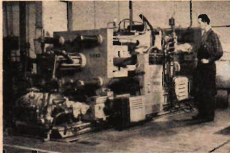
F. v.: Pressgjutningsmaskin, fabriken Cleveland, typ kalkkammare. Nedan: Detta är den största seriebyggda pressgjutningsmaskin som tillverkats — det finns bara en i Sverige. På översidan syns en påmonterad anordning för dragning av slider. Maskinen, fabriken Lester, är av kalkkammartypen.
