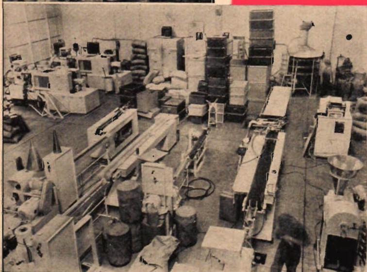
Överst t. h.: Kylarornament till Volvo gjuts i en mindre maskin. Detaljen, som är av zinklegering, ska sedan poleras och ytbehandlas. Därunder en smältuga med anordning för mekanisk beslekning. Nederst t. h.: Formsprutningsmaskin "Reed-Prentice" för plastdetaljer. T. v.: Formsprutningsmaskin, fabrikat Windsor.
