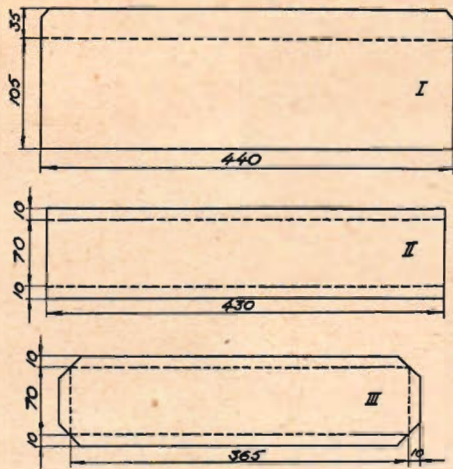
Fig. 1 (t. v.): Yttermåttarna på ramens delar. I är stöd för bildröret. II är gavlar. III är fram- och bakstycke, varav framstycket ska vara något kortare för att passa mellan gavlarna. Fig. 2 (nedan): Ramens delar med borrade hål. Fig. 3 (t. h.): Den färdigmonterade ramen.
