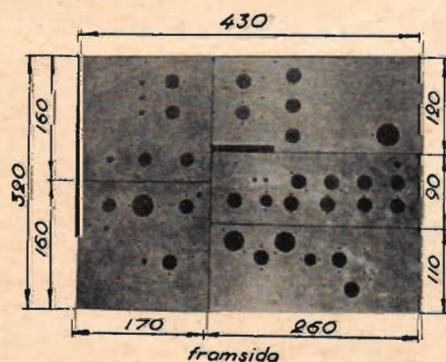
Fig. 4 (t. v.): Chassiplåtarna. Fig. 5 (t. h.): HF-enhetens chassi. Två plåtar klipps till, varav endast en borras. De bockas åt olika håll och kan därefter sättas ihop till en sluten låda.
