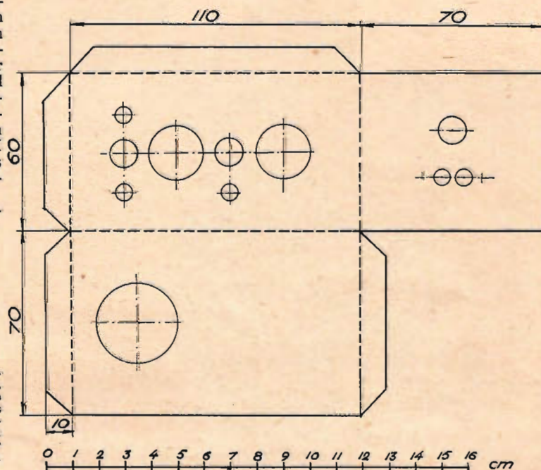
Fig. 4 (t. v.): Chassiplåtarna. Fig. 5 (t. h.): HF-enhetens chassi. Två plåtar klipps till, varav endast en borras. De bockas åt olika håll och kan därefter sättas ihop till en sluten låda.
