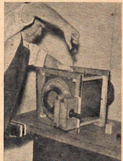
Stativet med 8 stödrullar till rälsen och pinjongaxeln med kullagren monterade i kraftiga träblock är här uppbyggt kring mjölkflaskan.
