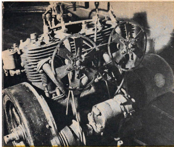
Motorn på en Phänomobil 1912 var luftkyld. Luften drevs bakåt av två fläktar. Bilen gick i Göteborg som droska på 20-talet, men förbjöds snart, då den gärna ville välta i kurvorna.
