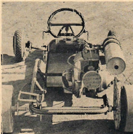
Prototypen var utrustad med en ILO LK 101 på 8,8 hk. Lägga märke till den enkla men effektiva skivbromsen.
