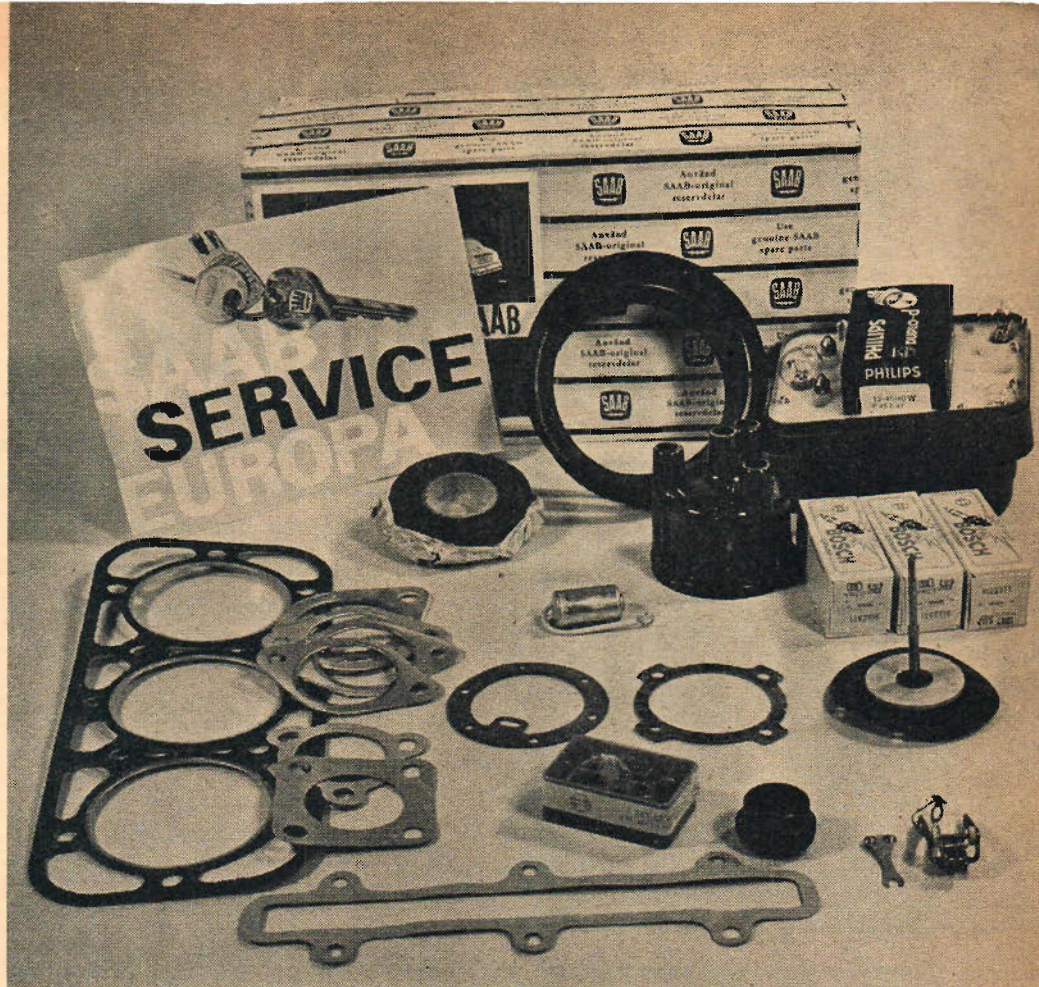
Reservdelsatsen för Saab kostar 100 kr och den innehåller följande: 1 motorpacksats, 1 vattenpumpspackning, 1 vattenpumpstättning, 1 packning för bränslepump, 1 membran för bränslepump, 1 brytarmekanism för bränslepump, 1 fördelarlock, 1 brytarsats för fördelare, 1 kondensator, 1 fläkträm, 3 tändstift, 1 lampetui, komplett med lampor och säkringar, samt 1 isolerband.
