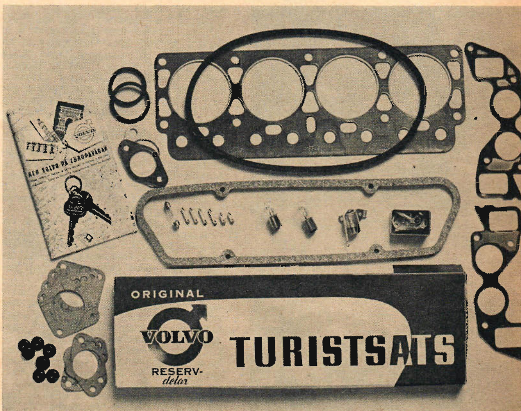
Innehållet i den reparationssats som Volvo tillhandahåller för 43 kr är: 6 säkringar, 3 glödlampor, 1 packning för bensinpump, 1 kondensator, 1 sats brytarspetsar, 1 packning för främre utblåsningsrör, 8 packningar för ventiler, 1 packning för ventilkäpa, 1 packning för cylinderlock, 1 packning för termostathus, 2 förgasarpackningar B 18 D, 1 förgasarpackning B 18 A, 4 förgasarpackningar B 18 D, 1 packning för in- och avgasrör och 1 fläkträm.
