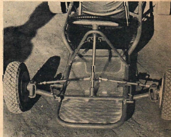
Star Kart är enkel att bygga men vi rekommenderar dem som inte har tillgång till egen verkstad att köpa ramen färdig. Kostar 170 kr.
