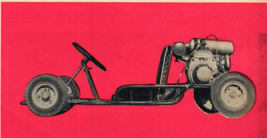
Detta är prototypen. Flera vagnar är nu färdiga för leverans och på dessa har bl a rattfästena flyttats längre bakåt och skumgummistoppad dyna finns nu också framför sätet.
