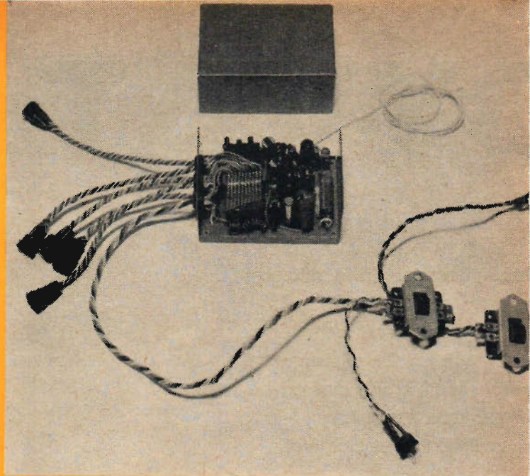
En reläös tiokanalsmottagare med transistorer. Plugg in-system för servon.
