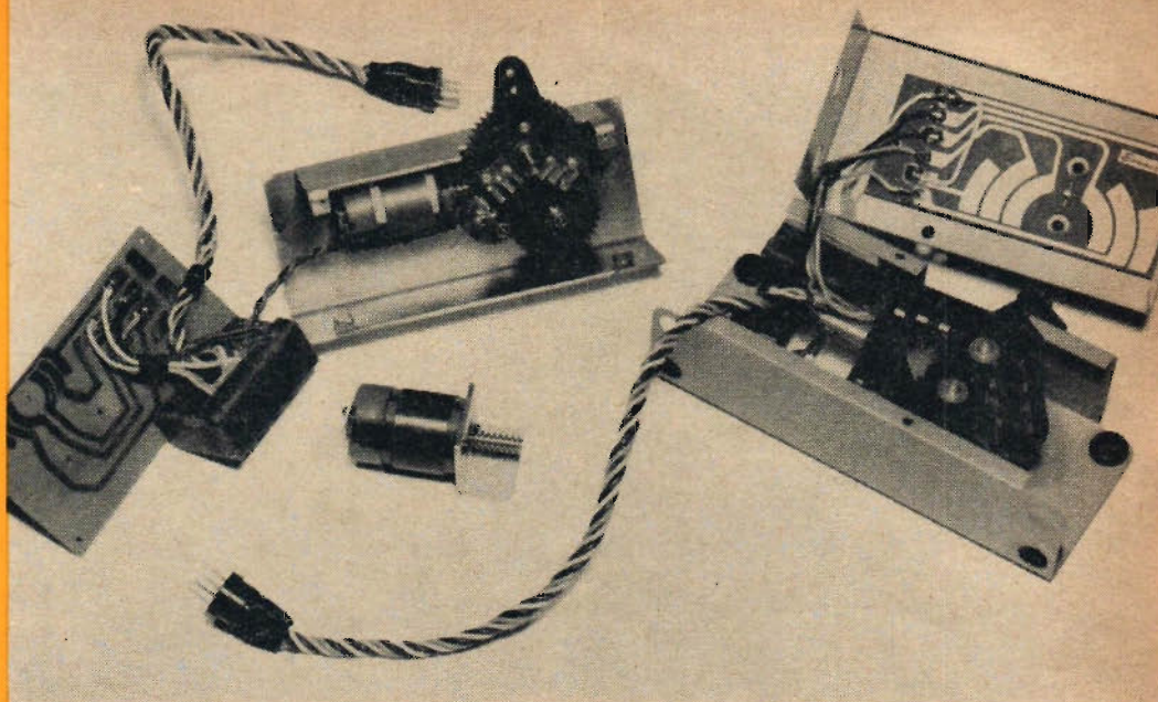
Bilden visar den tryckta kretsen för servistorn. Så installeras servistorn i Micromite- och Duramite-servon. Microperm-motorn har specialfäste för Micromite.
