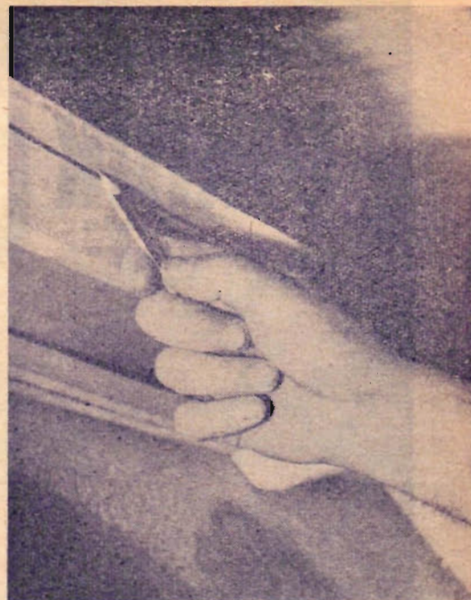
3 Plywoodborden är tilltagna med generös putsmän. Efter det att ett bord spänts fast på prov märks det upp för bortsågning av över-skjutande partier.
