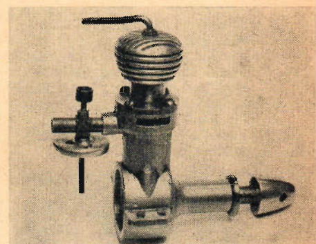
Gamla kända KOMET från Västerås.
