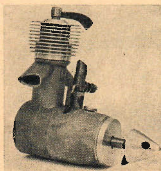
A5 — italiensk 5 cm 3 diesel från 1950.
