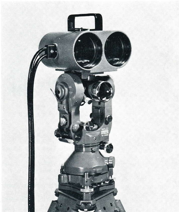
Teodolit Wild T2 med D1—10 T påmonterad
