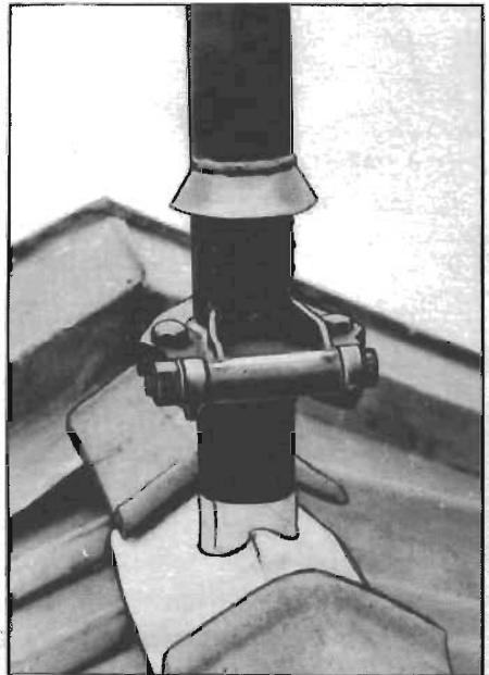
Bild 15. Fällanordningens ledningen
