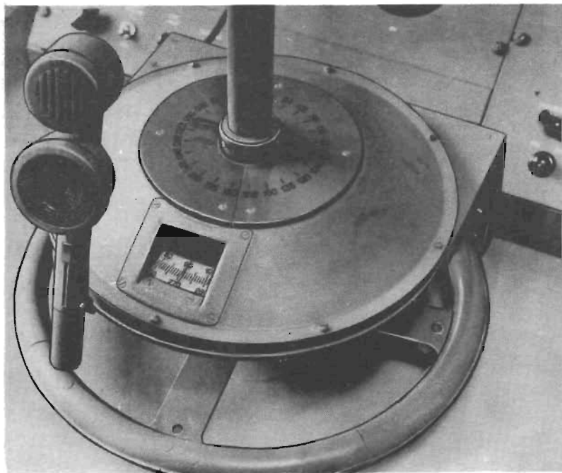
Bild 19. Mikrofonen samt pejlskalorna och orienteringsskalorna
