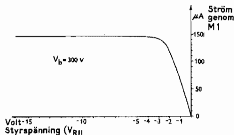
Bild 21. Strömkurva
