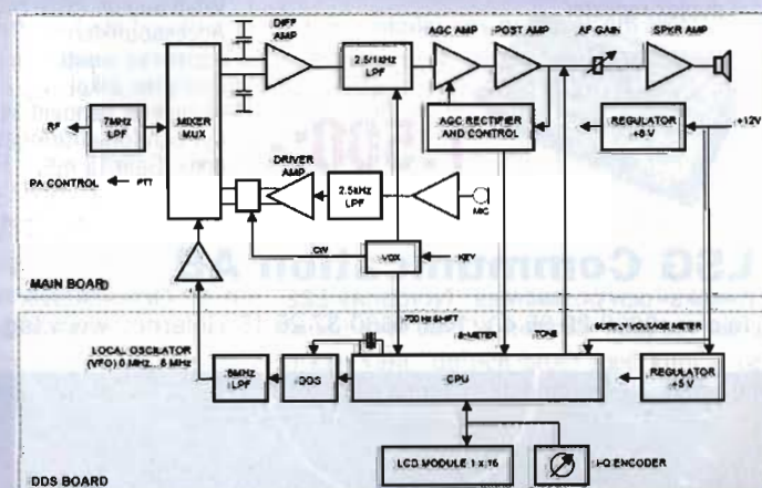
Blockschema till JUMA-TRX DSB/CW-rigg. Utifrån till vänster återfinns blandaren av typen 74HC4052.
