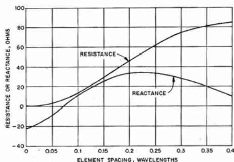
Fig. 4 Beräknad radiation resistance och reaktans hos direktorn som funktion av elements spacing då reflektorn är inställd för högsta möjliga gain enligt fig. 2
