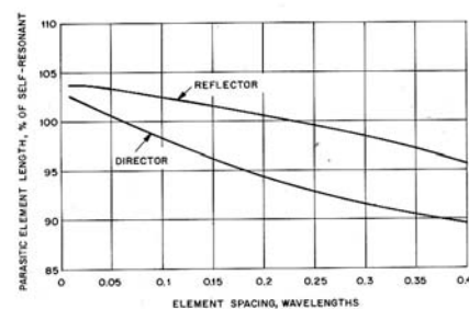
Fig. 3 Elementspadding i förhållande till ändring av elementlängd från självresonans för maximum gain.
