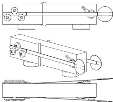
Bilden visar konstruktionen av manipulatorens. Plexiglasblocket har måtten 8×12×55 mm. Ritning gjord av Johan Eidenvall SM5XZB
