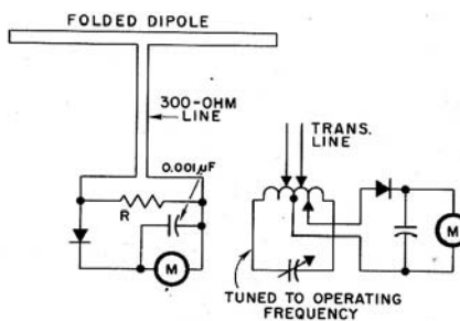
Fig. 5 Arrangemang med fältstyrkemeter. R bör vara ett non-induktivt motstånd på 300 ohm för bästa belastning för feedern. Om känsligheten inte räcker kan man använda den resonanskrets som visas till höger i figuren. Instrumentet kan vara en 0–1 milliampere meter eller ev. känsligare.
