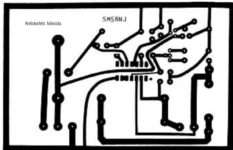
Överspänningsskydd med IC3423, inkopplat mellan A, B och C i kraftaggregatet och monterat under kretskortet.
