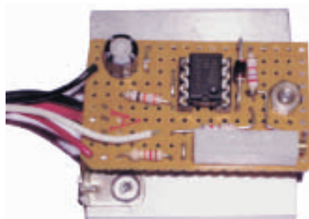
Överspänningsskyddet byggt på ett litet kort med tyristorn under kortet, klämd mot kylplattan.
