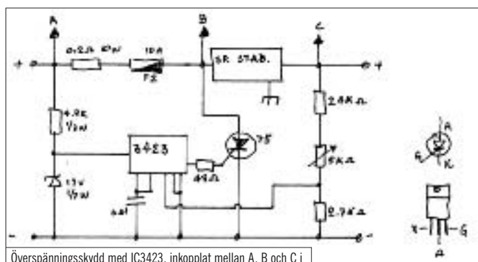
Överspänningsskydd med IC3423, inkopplat mellan A, B och C i kraftaggregatet och monterat under kretskortet.
