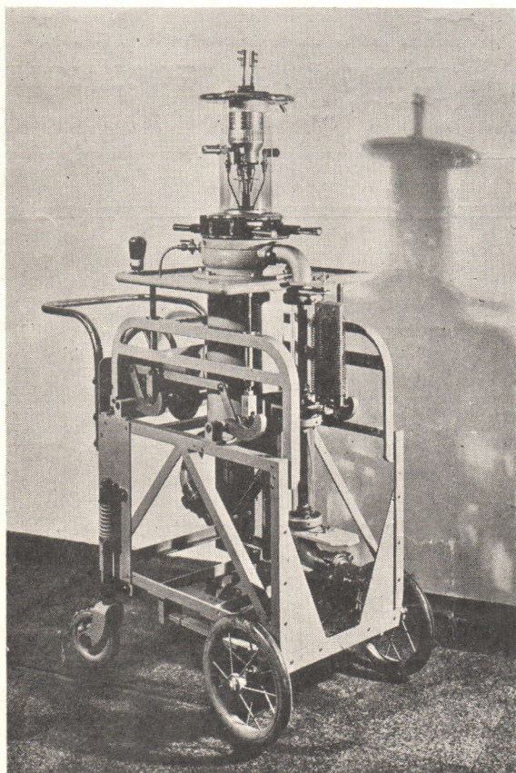
ETT SÄNDARRÖR AV DEN TYP, SOM KOMMER ATT ANVÄNDAS I DEN NYA MOTALASTATIONEN
