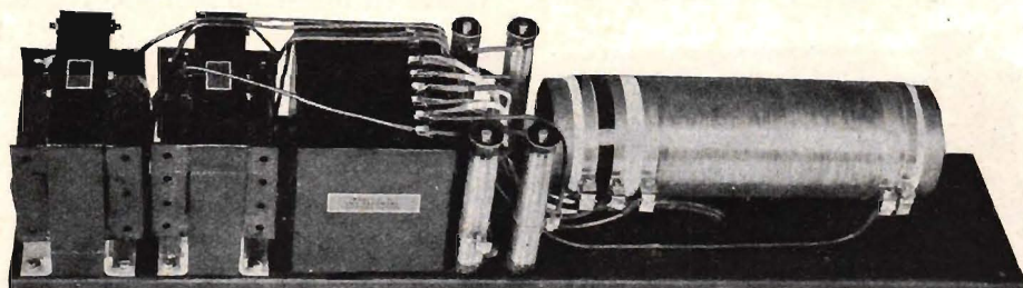
Fig. 5. Likströmsapparaten montage.
