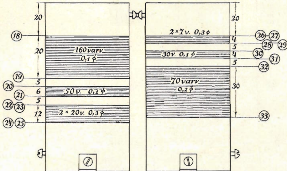
Fig. 4. Spolsystemet L_4 .
