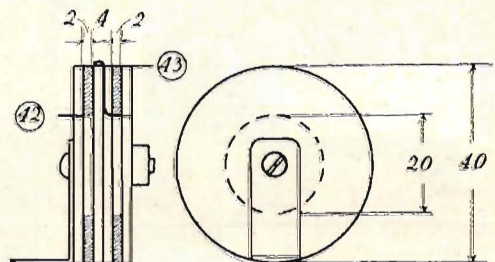
Fig. 7. Drosseln L_6 .
