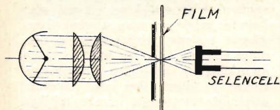
Fig. 3. Återgivningsanordning.
