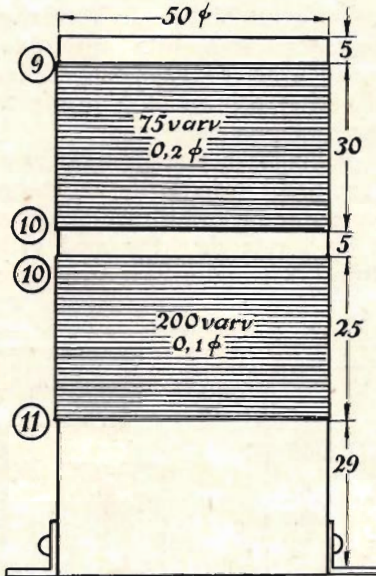
Fig. 2. Spolen L_1 .
