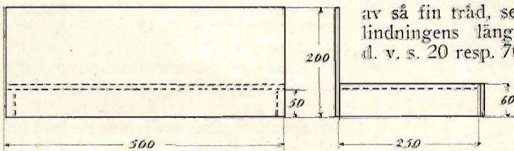
Fig. 8. Montageinnehållskonstruktion.
