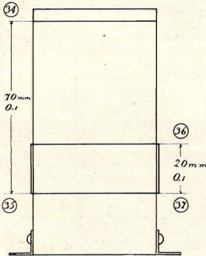
Fig. 5. Spolen L_4 .
