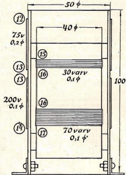
Fig. 3. Spolen L_2 .
