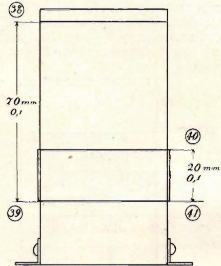
Fig. 6. Spolen L_5 .
