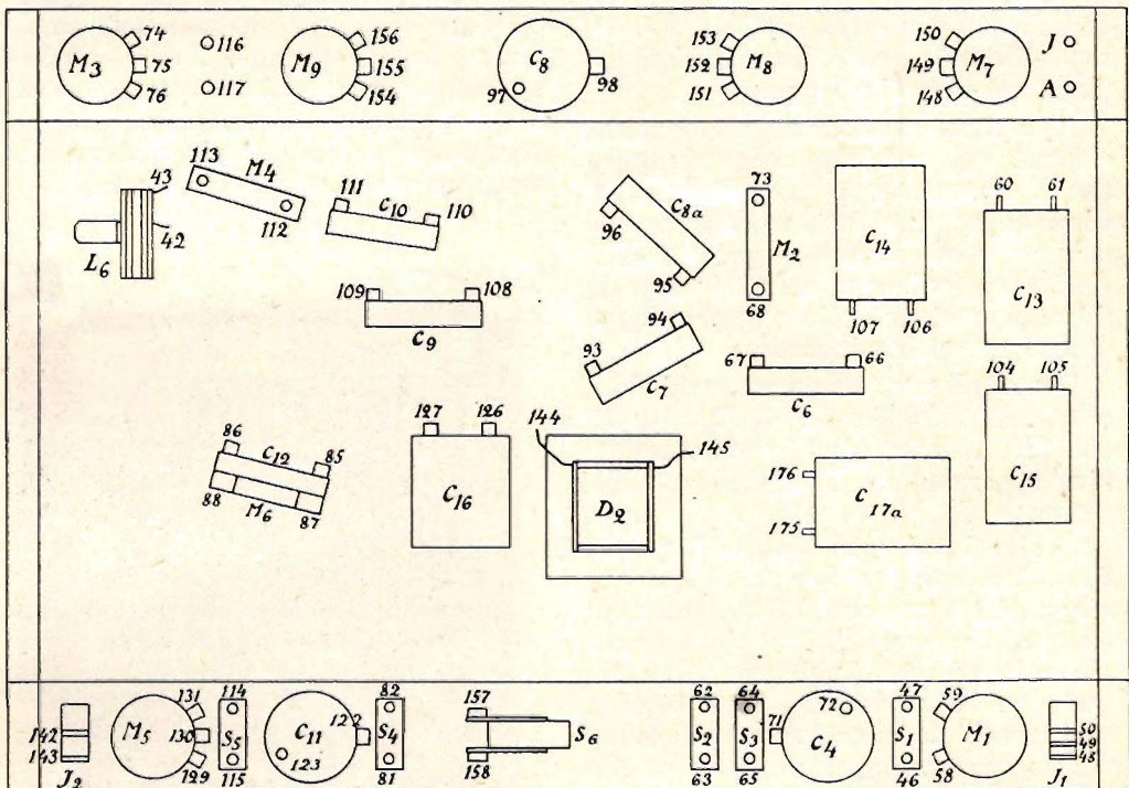
Fig. 9. Placeringsritning för mottagaren.
