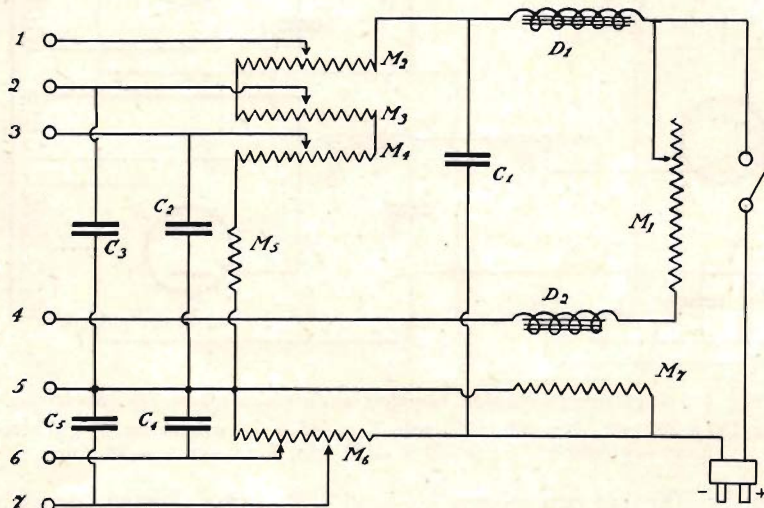
Fig. 4. Kopplingschema för nätanlutningsapparaten för likström.
