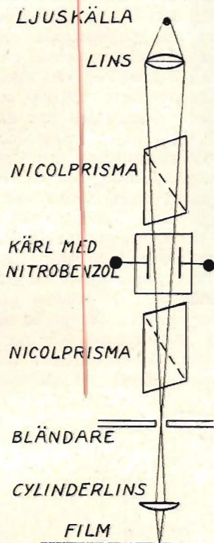
Fig. 1. Ljudregistrering med Kerrcell.
