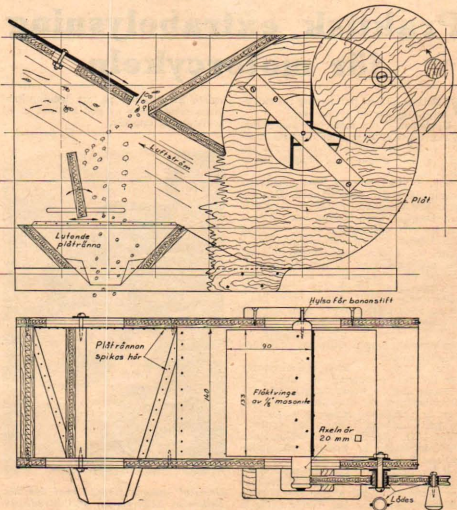
Ritning till lingonrensaren. Rutorna i övre ritningen har 5 cm sida.
