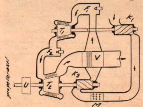
Fig. 4. Elliot-Lysholm gasturbin för fartyg.
