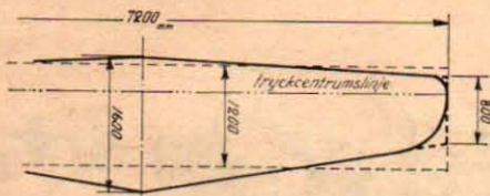
Fig. 7. Vinge.
