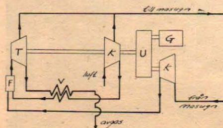
Fig. 7. Gasturbinanläggning vid masugn. K kompressor. T turbin. U utväxling. F förbränningskammare. G generator.
