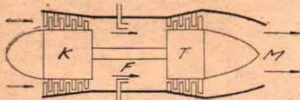
Fig. 1. Reaktionsdrift.
