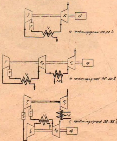
Fig. 3. Term. verkningsgrader vid 650° C. K kompressor. T turbin. F förbränningskammare. V värmväxlare. M mellankyllare. G generator.
