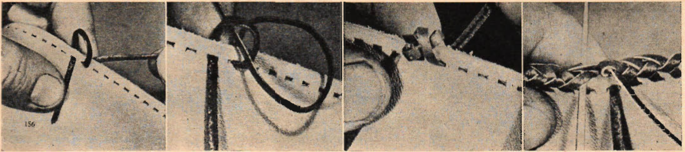
Fig. 5 (bildraden ovan): En av de vackraste snörningarna är den s. k. points de gause. Här gör man hälen med ett snett kort järn som gör en rak kort skära. Snörningen utförs på följande sätt: (1) Tråd enda änden av remmen genom ett hål. För remmen över kanten och stück in den i nästa hål (2). Tråd sedan remändan genom första öglan men se till att remmen går in från öglans vänstra sida. (3) Dra åt den första öglan och stück in remändan i nästa hål på så sätt att öglan korsas. Upprepa sedan samma sak. I hörn som måste vara rundade och försedda med ett hål mlitt i hörnet tar man två "styg" i samma hål.
