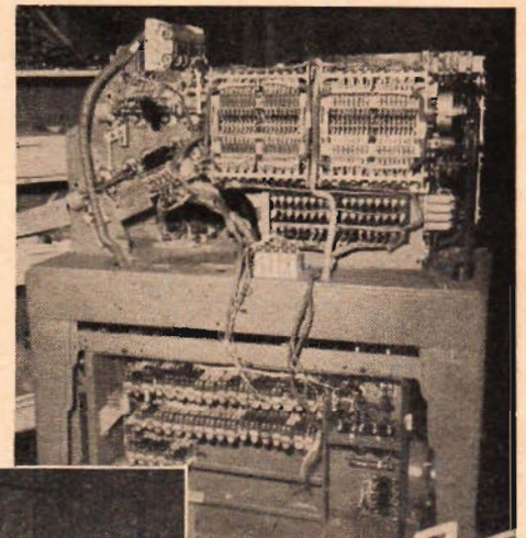
Ovan: Tabulatorn typ 416 under elektrisk montering.
