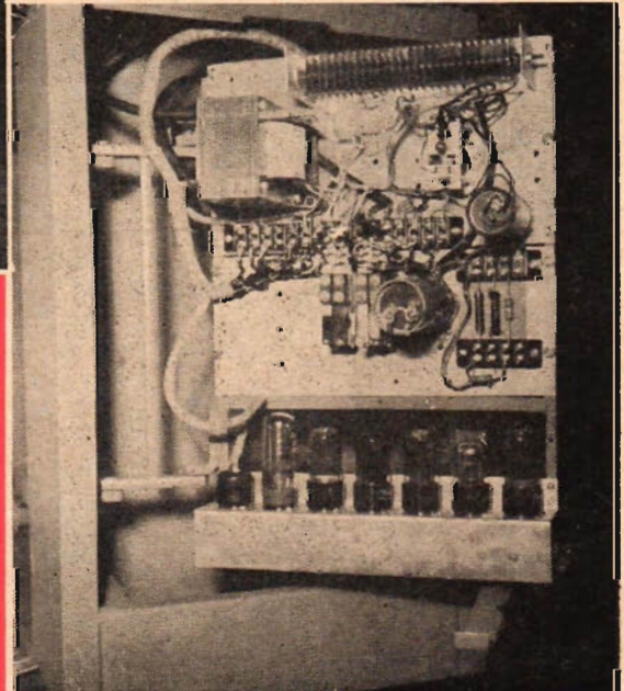
Ovan: Alfabetisk stansmaskin med relägrinden utfälld.
