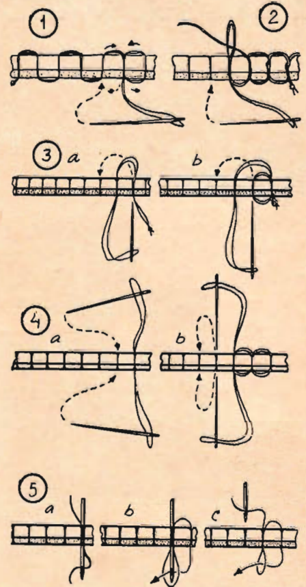
Fig. 3: Förstyng (1) är den vanligaste sömmen för läder och skinn och likaså sadelmakarsömmen (2). (3), (4) och (5) visar exempel på andra sömmar med stor styrka.
