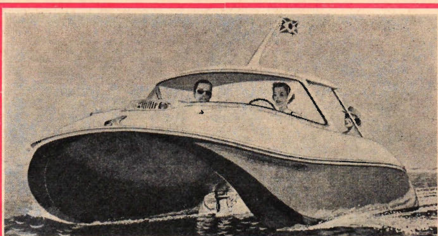
Båten är gjuten i plast och konstruerad efter bärplansprincipen med tydlig påverkan av polynesiernas katamaran-båtar. Den har en V-formad tvärsektion och vid full fart vilar endast de båda "medarna" mot vattenytan. Som syns på röntgenskissen på föregående sida täcks de tre motorerna av en huv som lätt kan svängas upp. Båttaket över förarplatsen är upp- och nedfällbart efter önskan och så som skissen visar. Utrymmet närmast framför motorhuv kan därigenom vid soligt väder förvandlas till en heltäckat liten kajuta.
