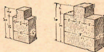
"Pilotattrappen", den "betalande lasten" har dessa mått i England och USA (2 v. för upp till 1,5 cc motorer, t. h. 3,5 cc. Måtten i tum.
