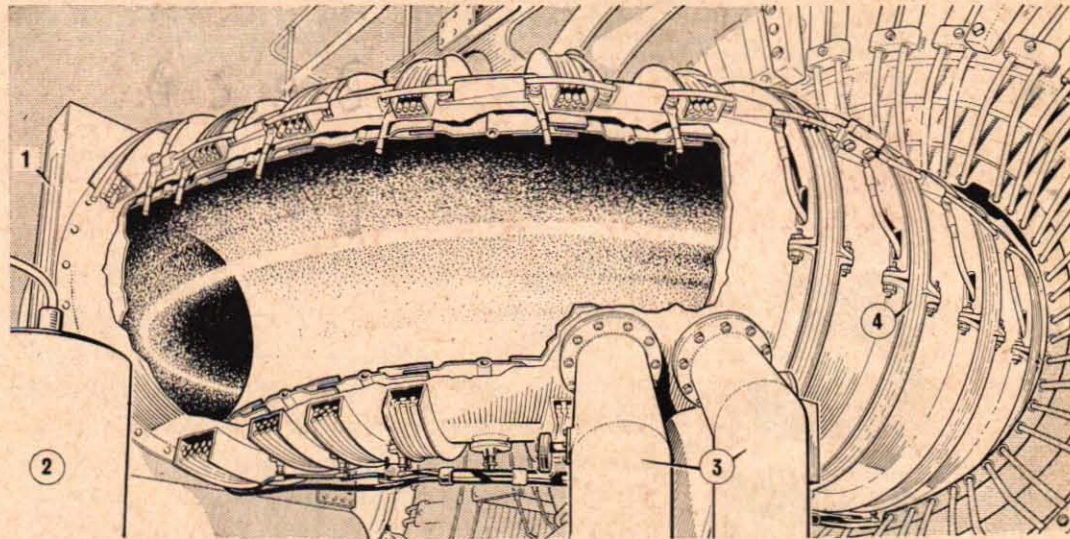
Siffrorna på denna röntgenteckning av urladdningsröret visar: 1 observationsfönster; 2 kylanläggning; 3 vakuumpump och 4 det axiala fältets spollindningar. Teckningen nedan visar några av de metoder som kommer till användning för att kontrollera processerna inuti det väldiga urladdningsröret.
