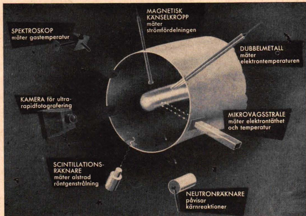
Siffrorna på denna röntgenteckning av urladdningsröret visar: 1 observationsfönster; 2 kylanläggning; 3 vakuumpump och 4 det axiala fältets spollindningar. Teckningen nedan visar några av de metoder som kommer till användning för att kontrollera processerna inuti det väldiga urladdningsröret.
