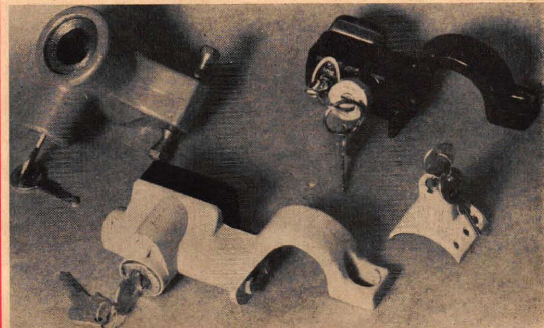
Rattlåset har, som framgår av namnet, till uppgift att hindra stöld genom att låsa rattet i ett visst läge. Liksom när det gäller växellåsen är de en tapp, som här är den hindrande detaljen. Fr. v. ses Wasos rattlås för Fiat 600, pris 85 kr, Neijman för Volkswagen, 85 kr inklusive montering, Huf, också för Volkswagen, 80—85 kr med montering, samt Nobb 80—95 kr med montering (går till alla märken).
