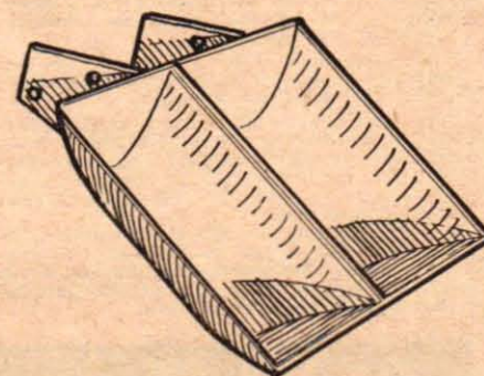
Vid flänsarna A fästs skovelarna med skruv. Fästöröronen B utgörs av trapezformade plåtbitar. De sneda sidorna lutar 15° från baslinjen.
