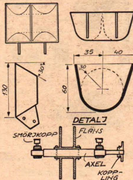
Fig. 3 visar turbin-skovelarnas dimensioner. Skovelarna fästs vid två flänsar som svetsas fast på ett rör som sedan i sin tur träns på axeln och fästs med koniska pinnar eller lämpliga skruvar.
