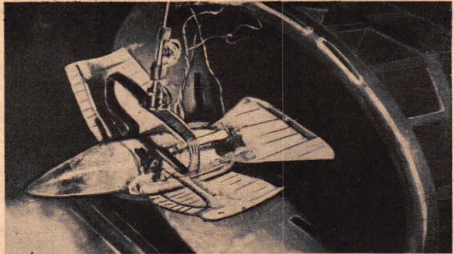
Ryssarna har bl. a. gjort omfattande vindtunnelprov med ornitopttrar, dvs. fågelvingade flygplan. Här testas en modell av ornitoptern OR-EM-3 i en vindtunnel. Den sensationella bilden har ställts till Teknik för Allas förfogande genom tillmötesgående av den ryska ungdomstidningen Komsomolskaja Pravda.
