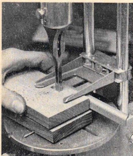
Borrstativet med borrstämtiltsatsen monterad. Den kan även användas till det kraftigare borrarstativet.
