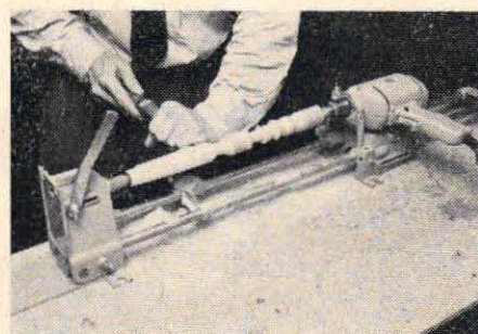
Svarvstativet är sammansatt av bänkstället TPLI (SA, motdocka) borrarstativsockel och försättare. Det hela sammanhålls av två stativstänger. Genom att "stjälpa upp" svarven vid motdockans led förvandlas den till bormaskin. Bänkstället är även grundstomme i andra kombinationer.
