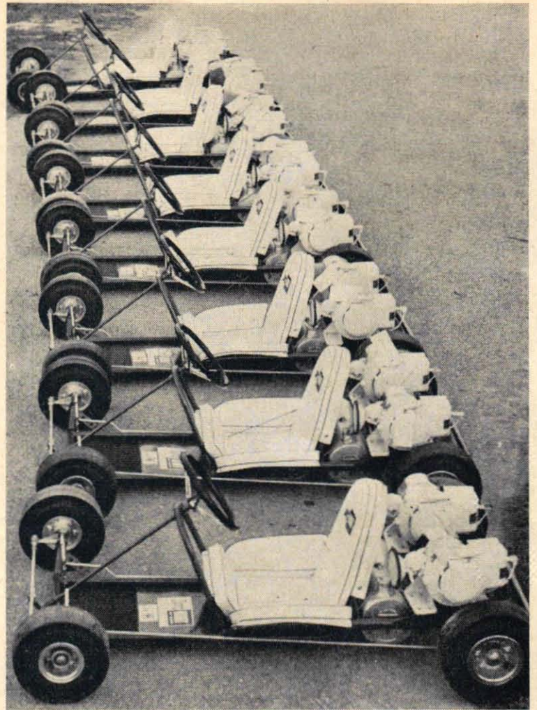
En del av de först importerade Dart-Kart-vagnarna. Samtliga är utrustade med släta däck, s.k. slicks, men om så önskas utbyts dessa utan extra kostnad mot mönstrade däck. Med två motorer kostar vagnen 2399.—.
