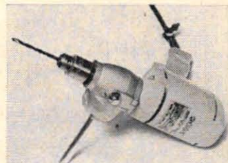
Till Bridges finns två typer av reduktionsväxlar. Bilden visar modellen som man med ett vred ställer på "fullvarv" eller reducerat varvtal.
