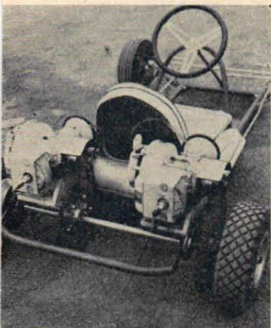
Tecumseh-motorerna på 95 cc utvecklar ca 6 hk vardera vid 8000 v/min. De driver direkt på den genomgående bakaxeln. 76-kuggsdriv är standard, men det finns drev i storlekar från 68 till 92 kuggar.
