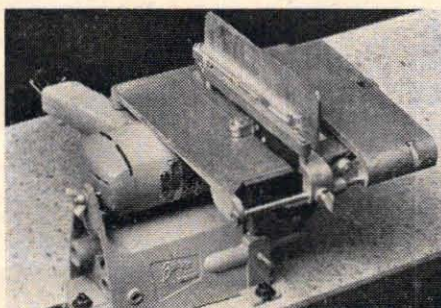
Bridges tappningstillsats byggs upp på det vanliga cirkelsågbordet. För upptagning av tapphålen används en annan tillsats, som monteras på svarvens motdocka. Tappningstillsatsen fungerar tillfredsställande, så när som på att monteringen av cirkelsågbordet faktiskt är ganska besvärlig.
