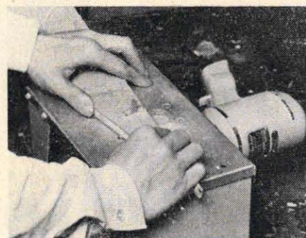
Genom att kombinera kontursågen med bänkställ KB/SA3 får man en utmärkt bänksticksåg. Ett antal blad för olika material som plywood, masonit, asbest, bakelit, aluminium, etc. finns att få.
