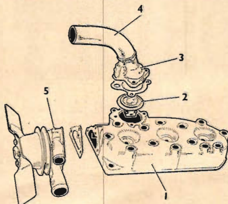
Omkonstruktionen av SAAB-motorns kylsystem innebär att vattenpumpen och termostaten är placerade direkt på motorn cylinderlock. 1. Cylinderlock. 2. Termostat. 3. Termostathus. 4. Slang till kylaren. 5. Vattenpump med fläkt.
