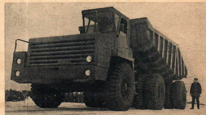
Bilen på bilden ovan tillverkas i Ryssland. Den lastar 65 ton och väger 27 ton. Fabrikket är Dumper Belaz-540. Byggs i olika modeller. Detta är den minsta.
