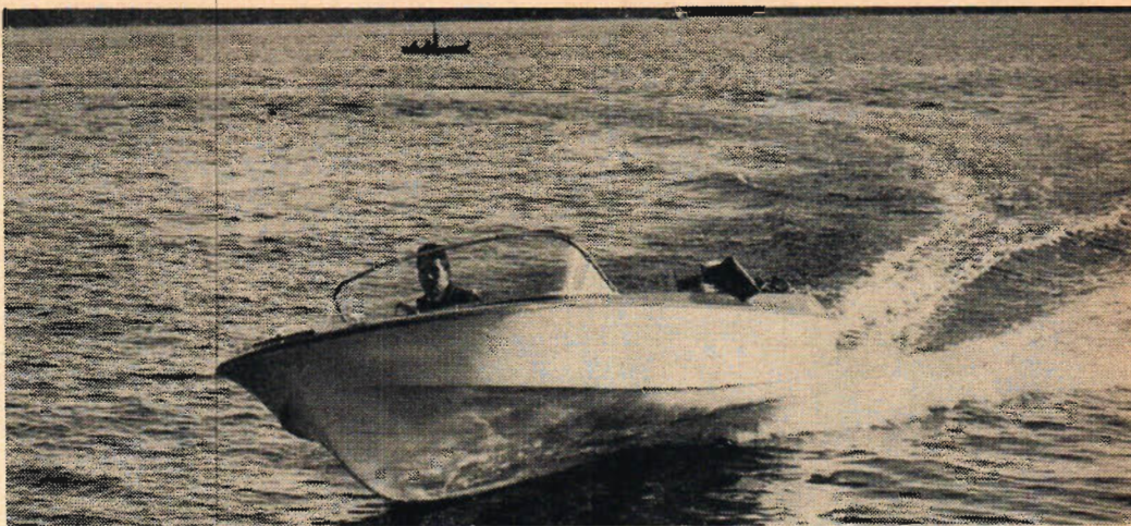
Herwa Star har en högt uppdragen slaglinje i fören och en botten med "klinklinjer". Båten planar lätt upp men tar lätt över sig ryksjö vid grövre motsjö på grund av den högt uppdragna slaglinjen.
