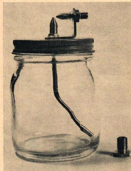
Modell Mini levereras utan slang för handblåsa eller fotpump. Den lösa delen till höger sätts på när man har en anslutning med större diameter. Behållaren rymmer ca 1,5 dl.
