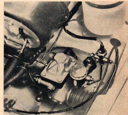
1965 års SAAB har hydrauliskt manövrerad koppling. Här visas de båda cylindrarna för kopplingen och för 2-kretsbrömsarna. De har, tack vare att bilen nu har hängande pedaler, kunnat placeras högt och lättåtkomligt.
