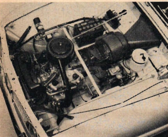
Motoreffekten i 1965 års SAAB är höjd till 44 hk. Kylsystemet är omkonstruerat så att kylaren är placerad framför motorn. Längst till höger på bilden syns den nya värmeanläggningen, som har avsevärt högre kapacitet än i tidigare modeller.
