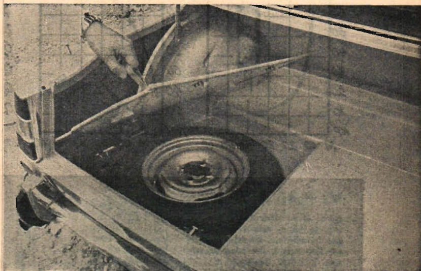
Bagageutrymmet är mycket brett tilltaget, det sträcker sig också långt in. Reservhulet sitter monterat under golvet. Detta arrangemang stjälar en del av djupet.
