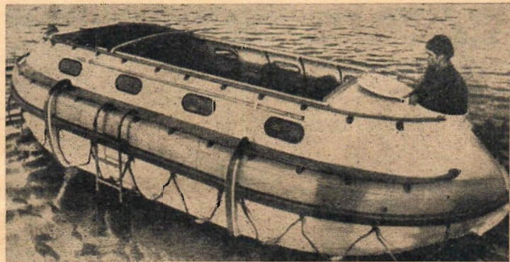
En ny livbåtstyp av glasfiberarmerad plast, Nicolboat, byggs nu i Norge. Som syns på bilden ovan ger den de nödställda gott skydd även i hög sjö. Ett tyskt skeppsvarv har redan beställt 32 sådana livbåtar.
