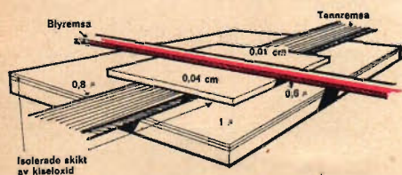
Kryotron bestående av två korsande, smala metallband. Det undre är av tenn, det övre av bly. De är elektriskt isolerade från varandra av ett tunt skikt kiseloxid.
