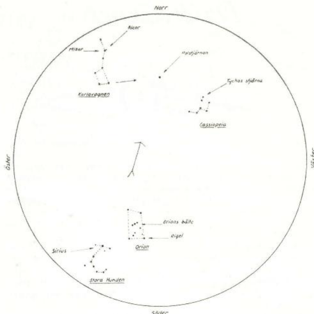
Några stjärnbilders lägen. December kl. 23—24. Observera vädersträcken.
