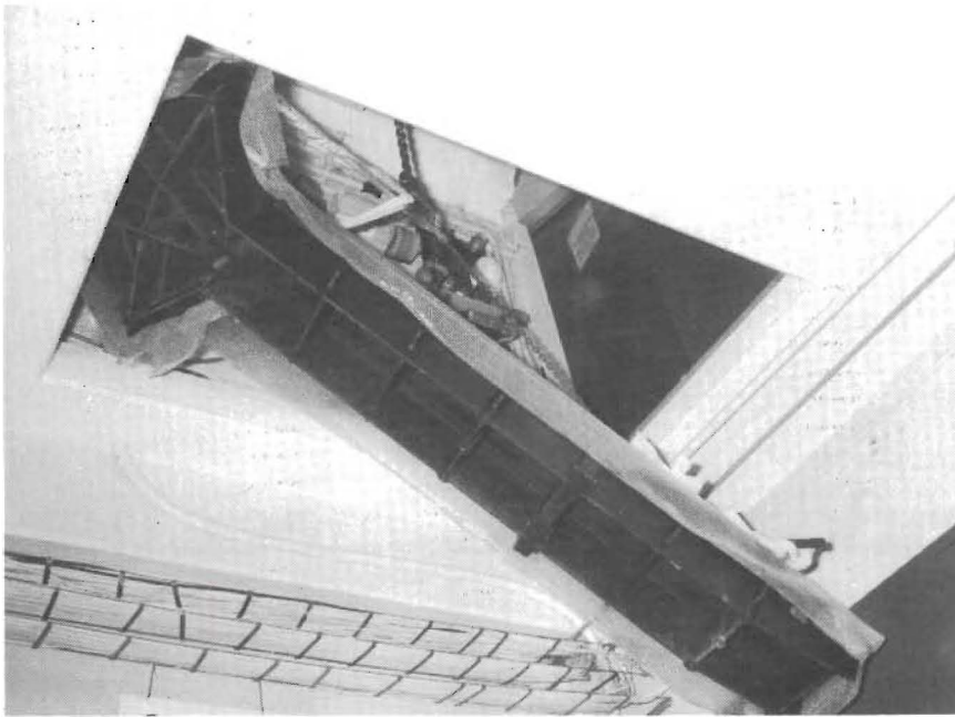
En optisk bänk måste vara absolut plan. Därför fick man ta till nya grepp för att sätta den "lilla fransyskan" på plats. Denna del väger omkring 1,5 ton.
