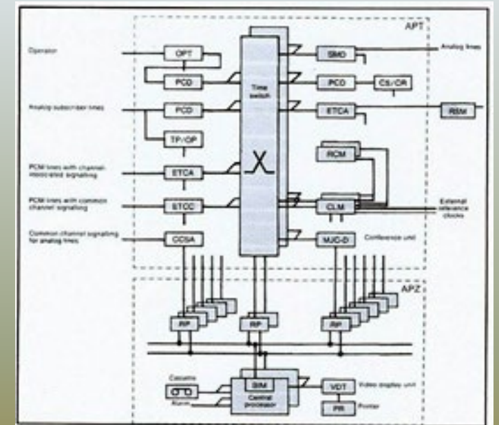
AXT-121 blockschema
