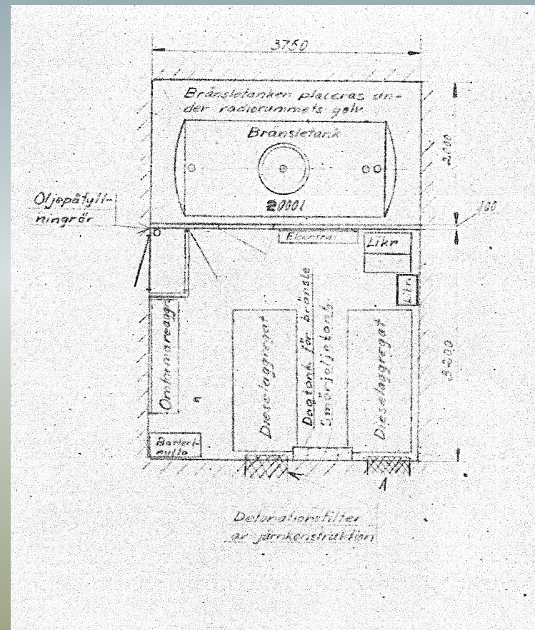
Elkraftinstallation
