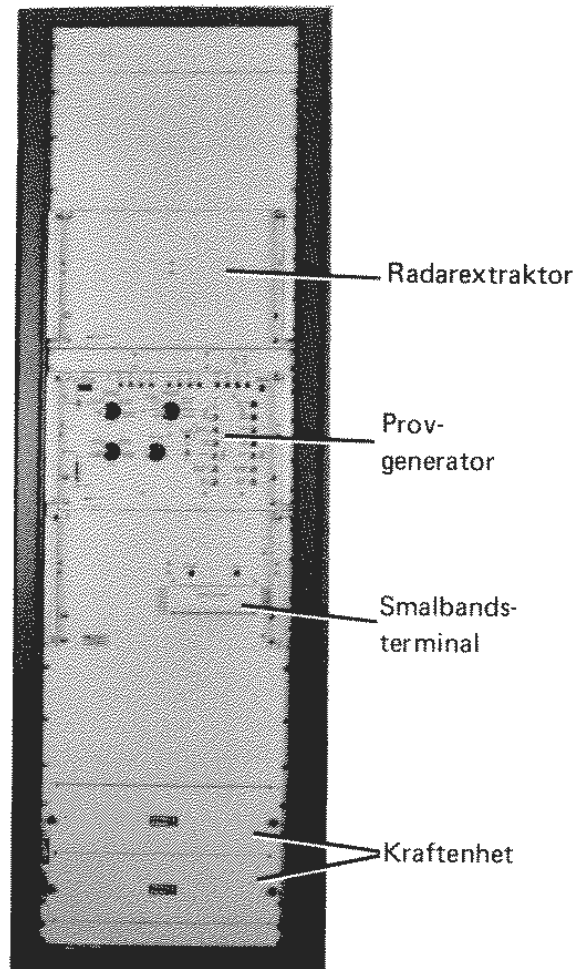
Bild 7. Datatransmissionsutrustning 109
