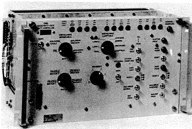
Bild 11. Provgeneratoren sedd framifrån.
