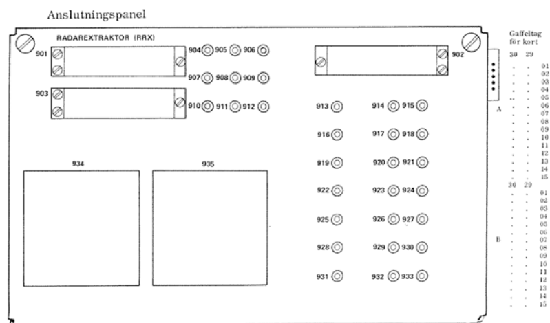
Bild 9. Radarextraktorns mekaniska uppbyggnad.
