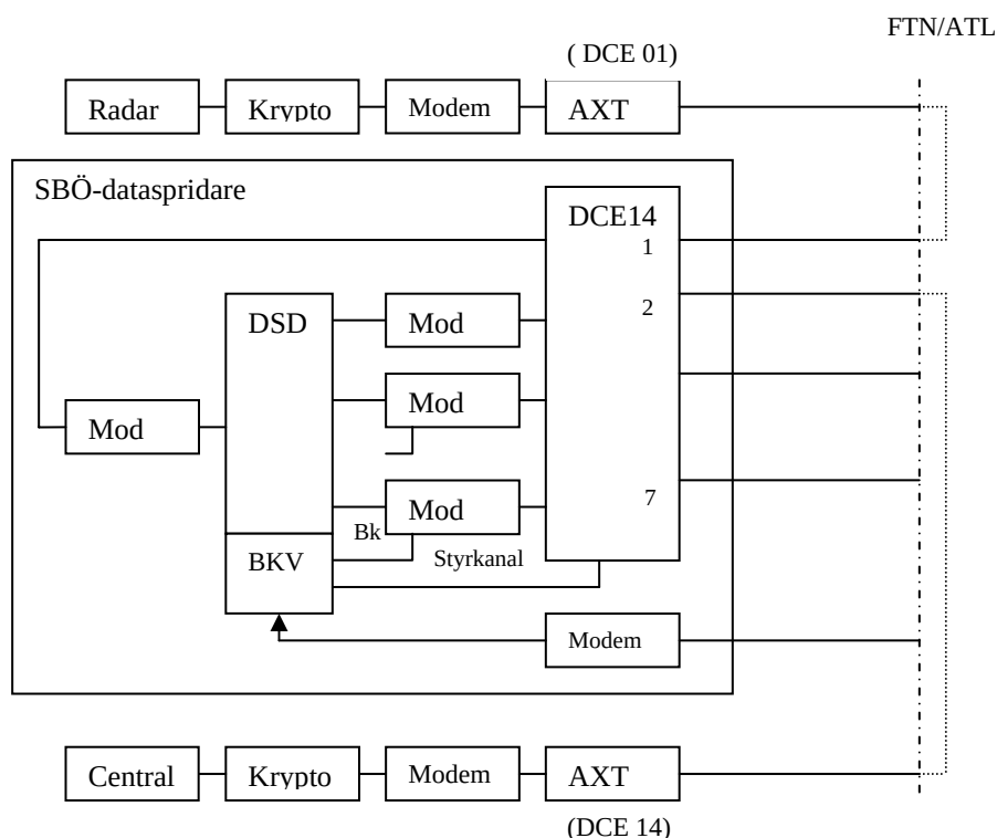
Fig 2.2 Principuppbyggnad av förmedlad SBÖ.
