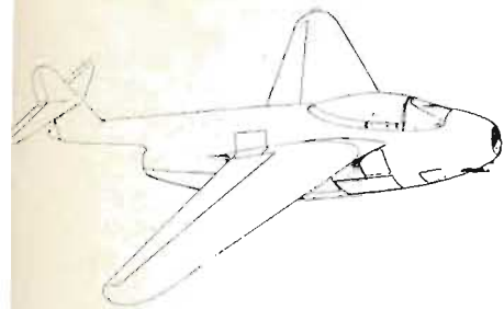
Ovan. Första skissen av J 29:an — som projekt kallades den då, 1945, för "R 1001". ■ Nedan. Vid utprovningen av den nya plivingsformen användes en SAAB 91 A Safir — med vingar i halvskala.
