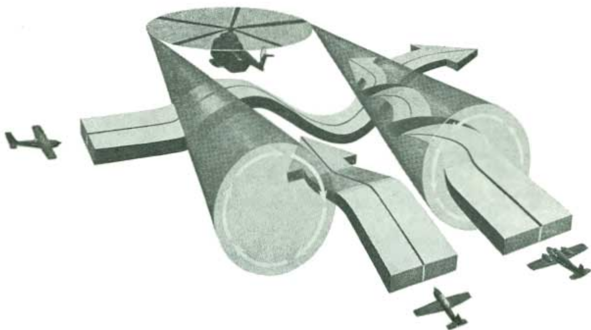
● Bilderna i v och nedan visar helikopters rotorbladsströmningar bildande ändvirlar med centrerad nedåtriktad verkan.
