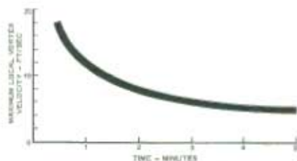
● Exemplet på en hkp:s kvardröjande luft-hastighet (ft/sek) hos ändvirlarna i förhållande till tiden.
