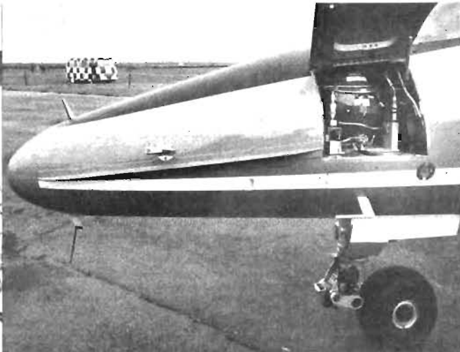
● Den franska 'AlphaJet'-versionen har framtill på nosen två långsgående, små 'fenor', som möjliggör för flygeleven mjukare/behagligare träning i spinnmomenten.
