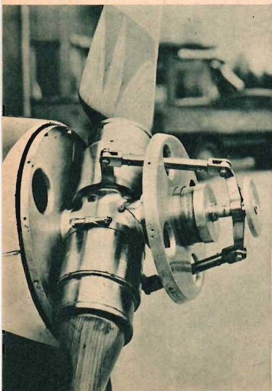
Principschema över Dynamicpropellern. De numrerade detaljerna är: 1) servocylinder, 2) kraftkolv, 3) hävarm, 4) stötsång, 5) regulatorkolv, 6) regulatorkolvstång, 7) luftplatta, 8) regulatorfjäder. — T v har spinnern tagits av och det slurriga navet ses oklätt med luftplattan längst till höger.
