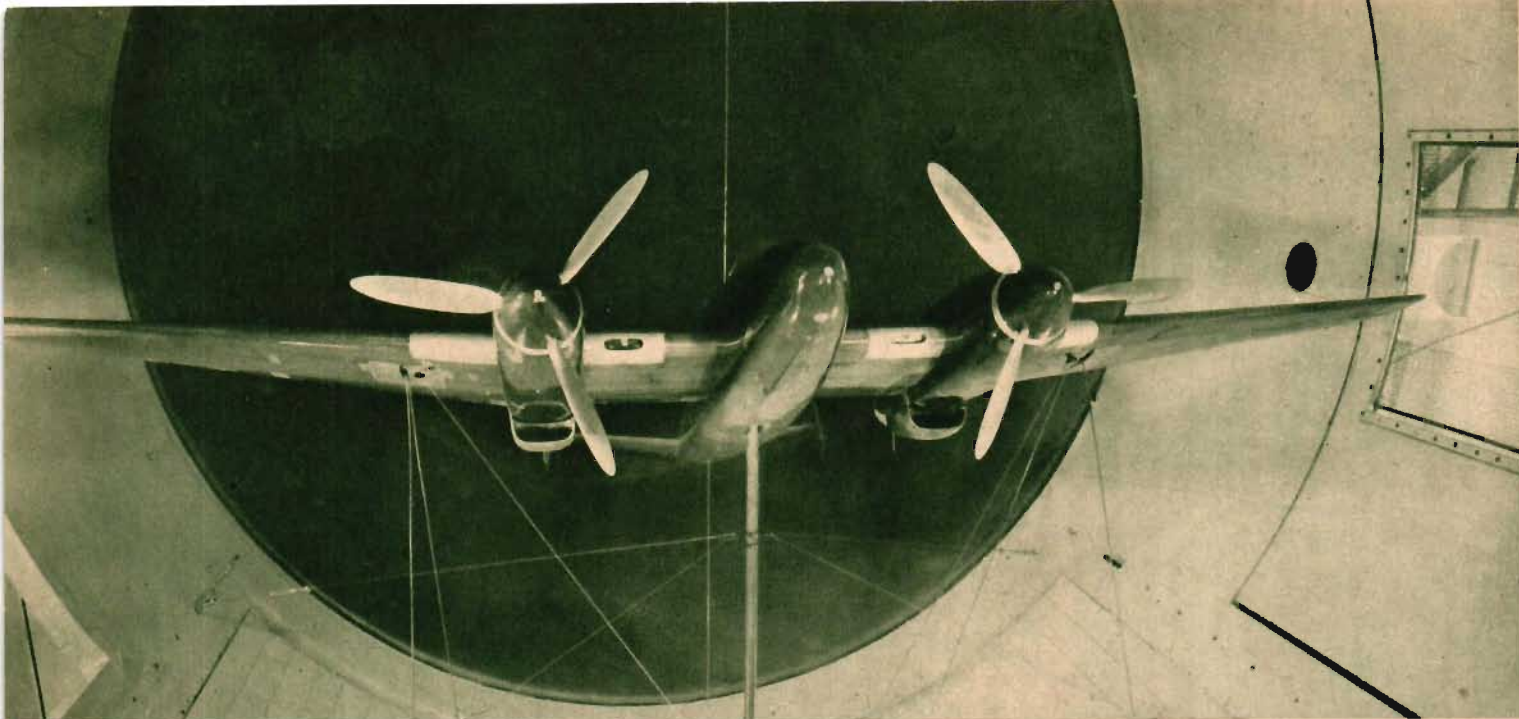
Den stora vindtunnelmodellen — 2,5 m spännvidd — till SAAB-24 »den svenska Mosquito» under prov med löpande propellrar vid flygtekniska försöksanstalten i Ulvaunda. De ytterst noggranna vindtunnelproven gav mycket goda resultat.
