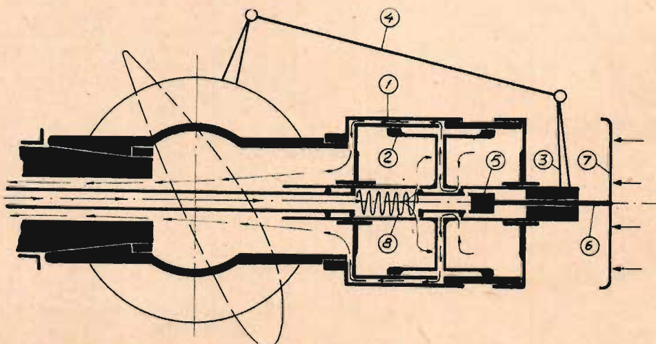
Principschema över Dynamicpropellern. De numrerade detaljerna är: 1) servocylinder, 2) kraftkolv, 3) hävarm, 4) stötsång, 5) regulatorkolv, 6) regulatorkolvstång, 7) luftplatta, 8) regulatorfjäder. — T v har spinnern tagits av och det slurriga navet ses oklätt med luftplattan längst till höger.
