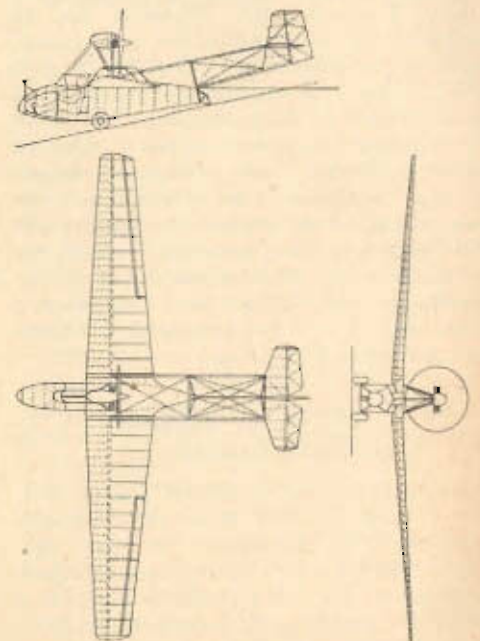
Översiktsritning.
