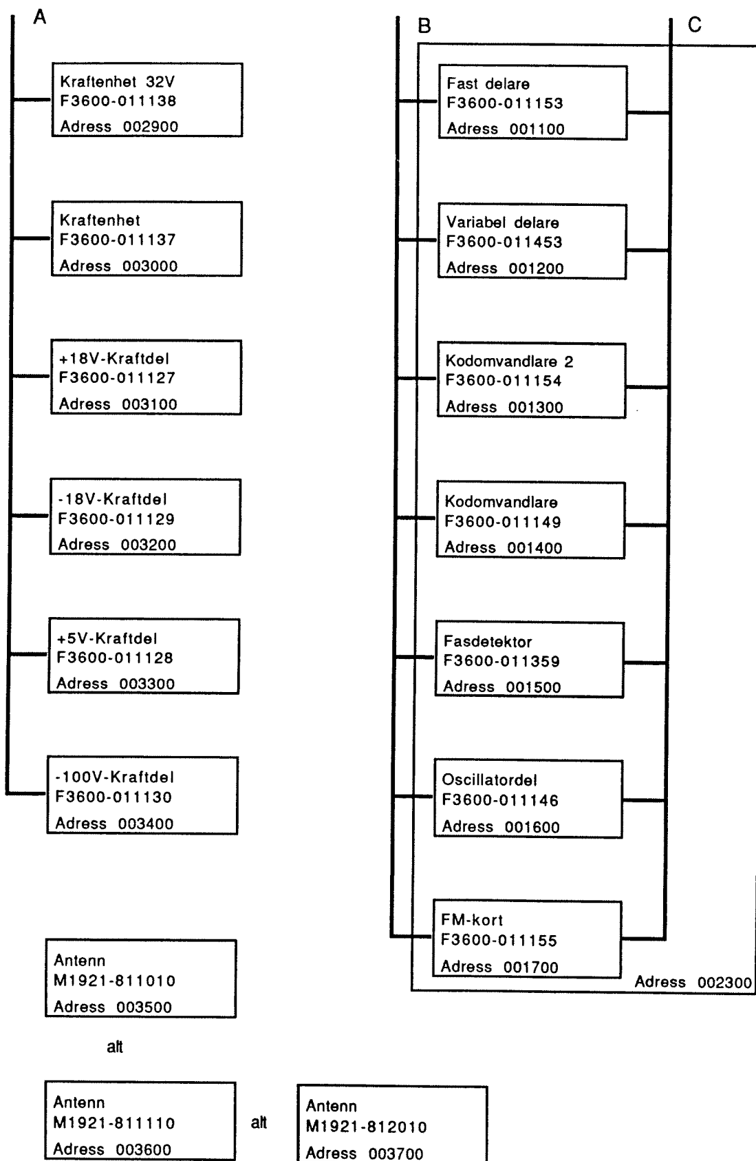
Blockschema RA 730
