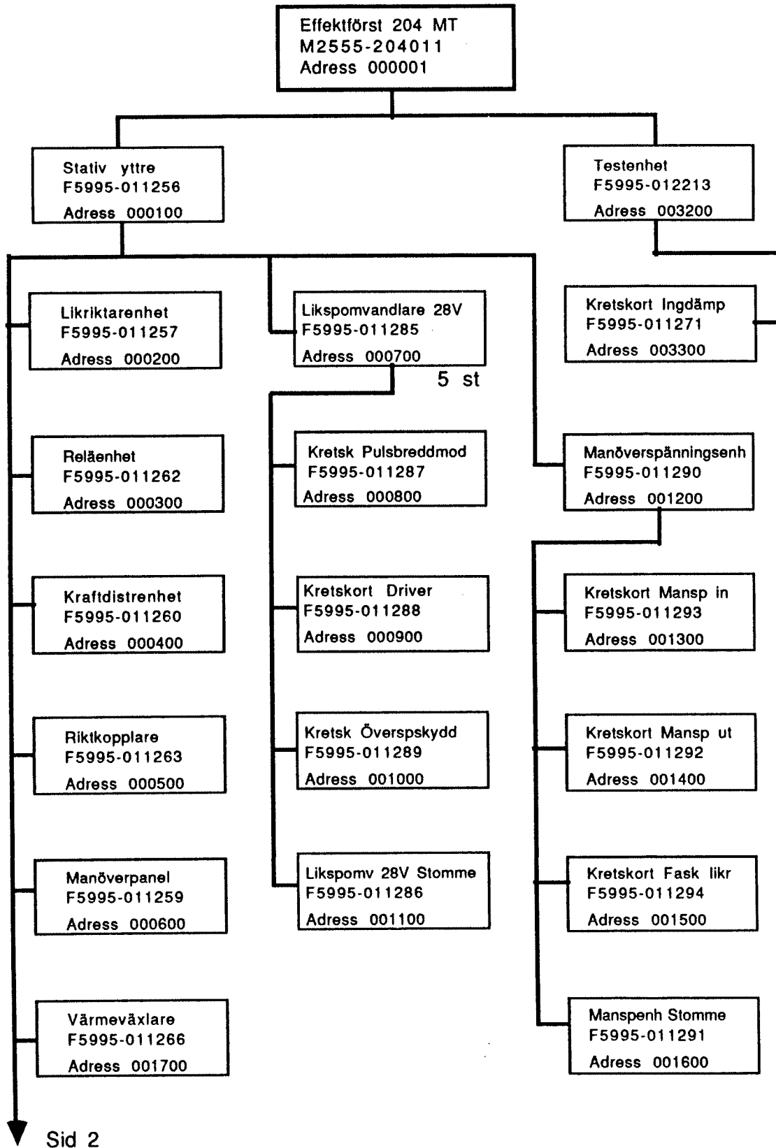
Blockschema effektförstärkare 204 MT
