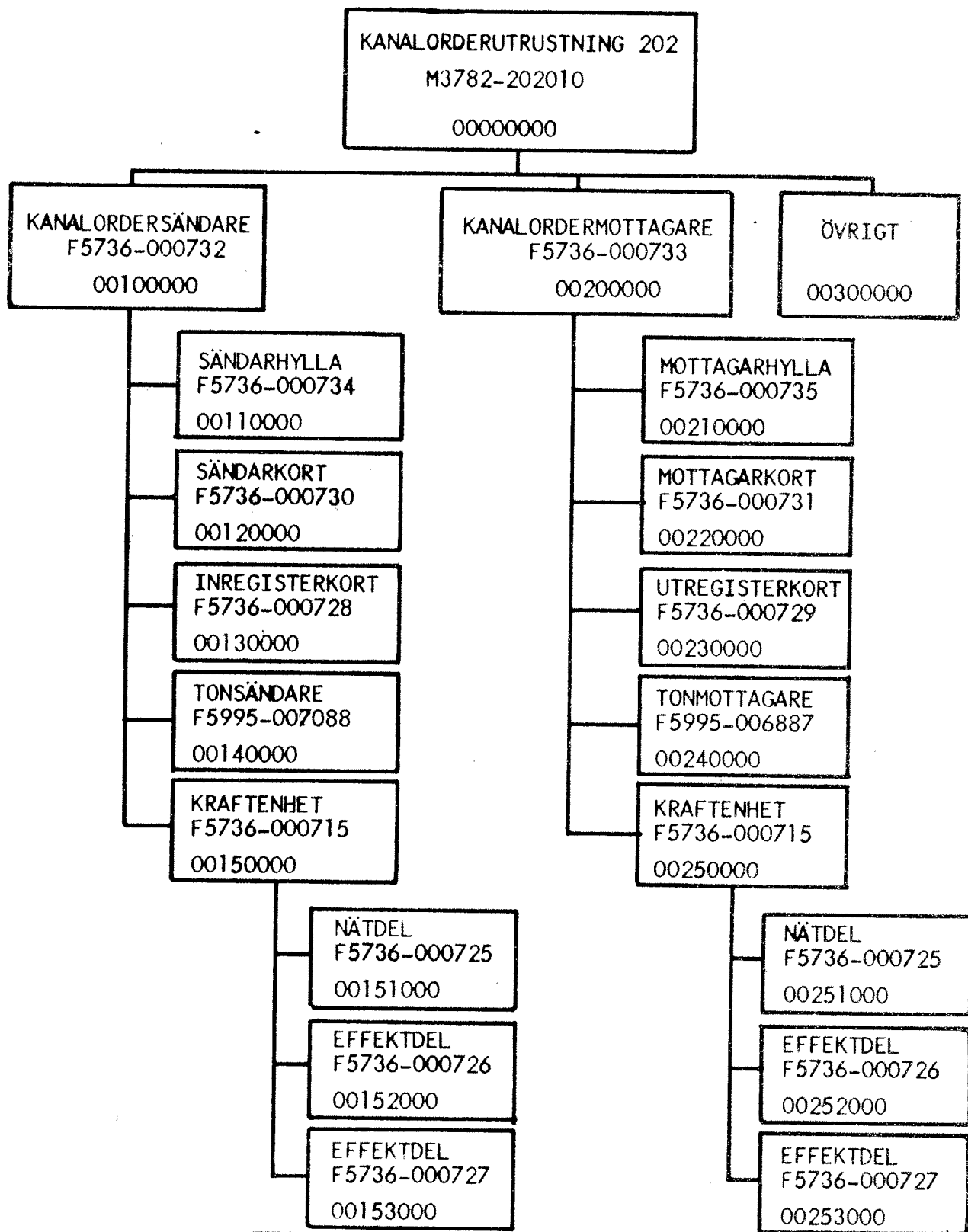
Bild. Kanalorderutrustning 202A Blockschema för Underhållsplan Apparater
