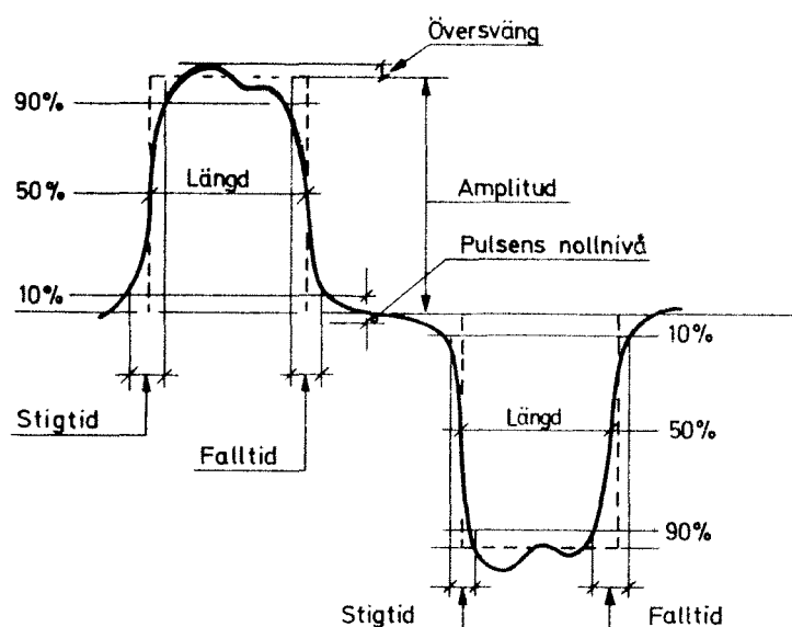
Bild 8. Pulsform 34 Mbit
