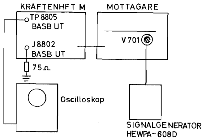
Bild 10. Uppkoppling, mottagarsidan
