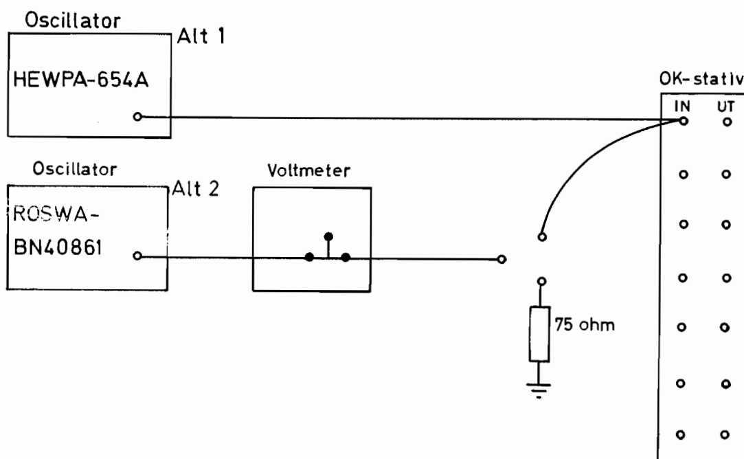
Bild 4 Uppkoppling, sändarsida
