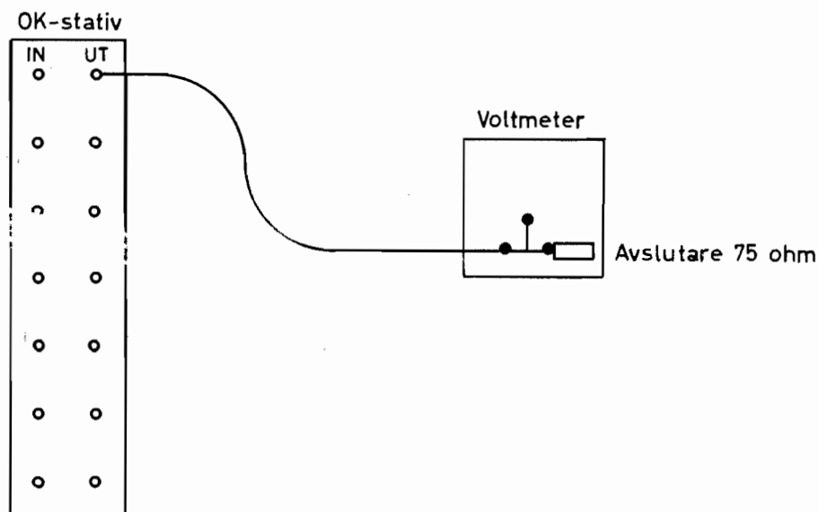
Bild 5 Uppkoppling, mottagarsida
