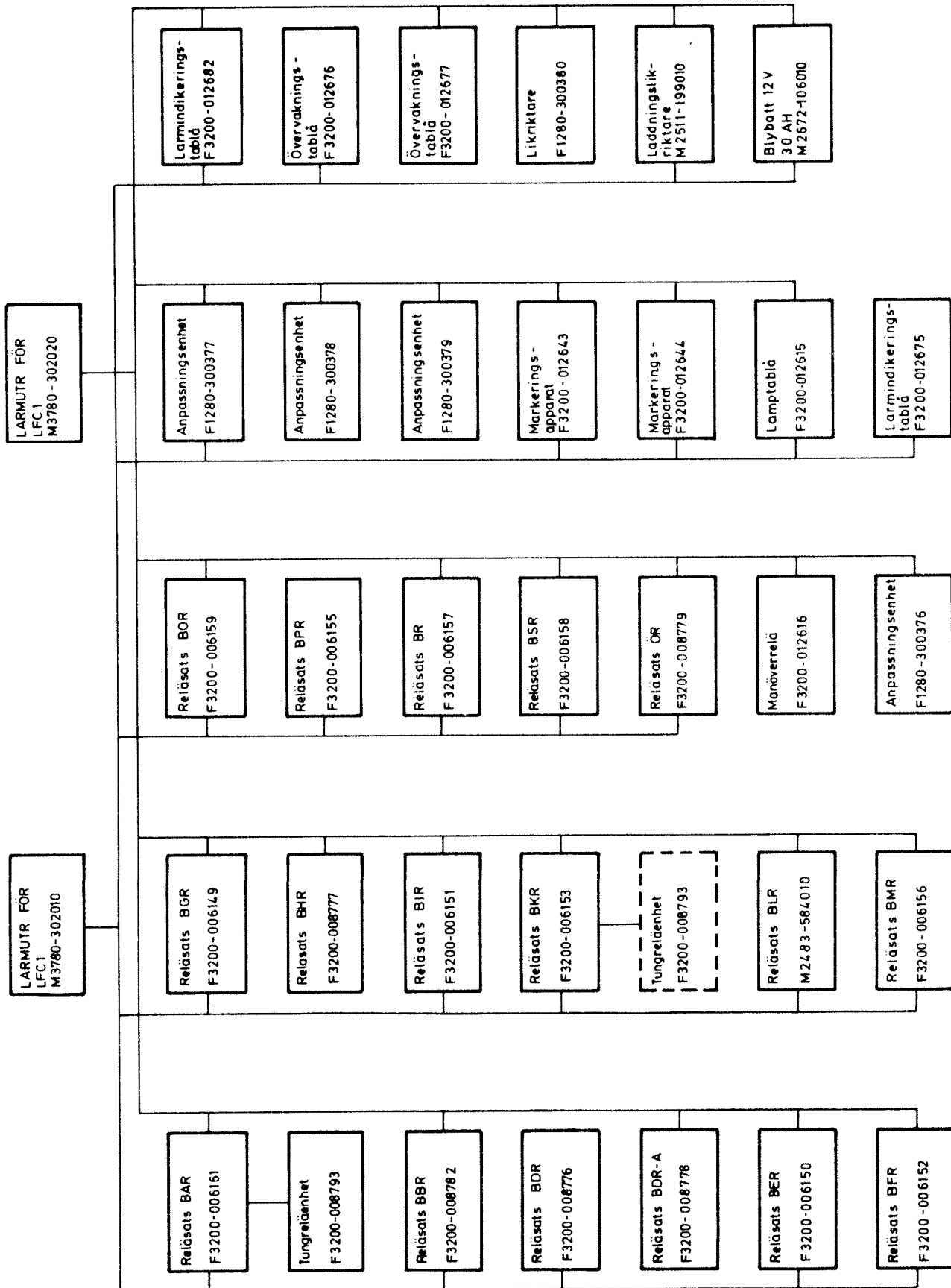
Blockschema för larmutrustning Lfc 1.
