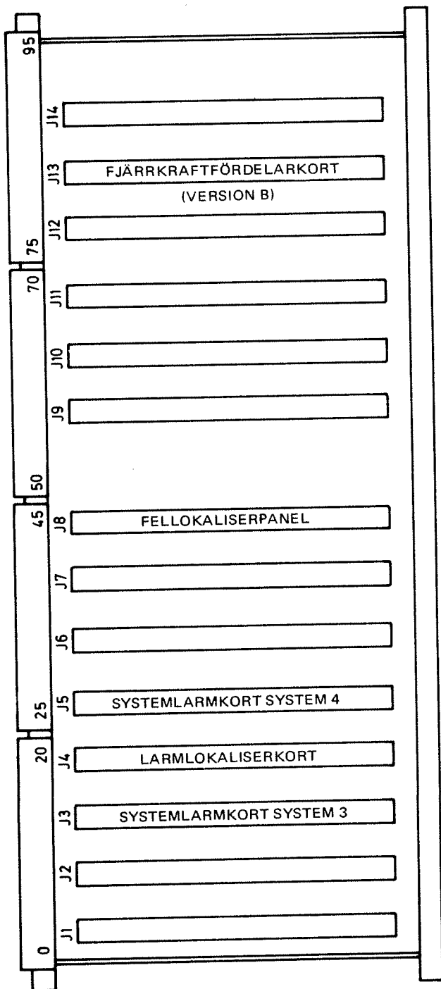
Bild 3. Larm och övervakningshylla
