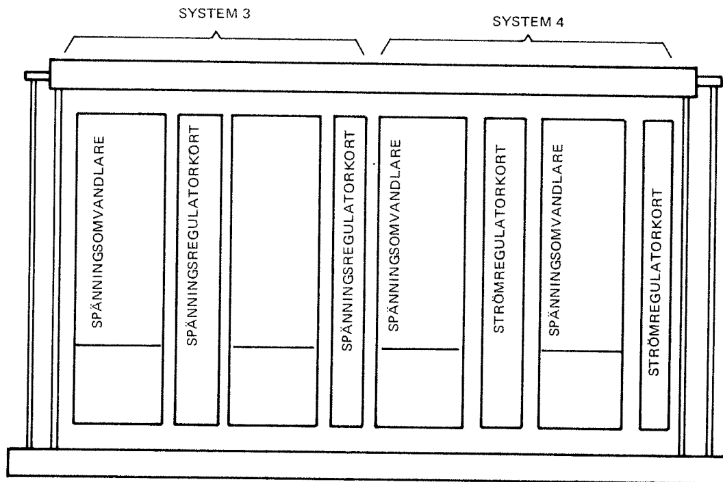
Bild 5. Kraftmatningshylla
