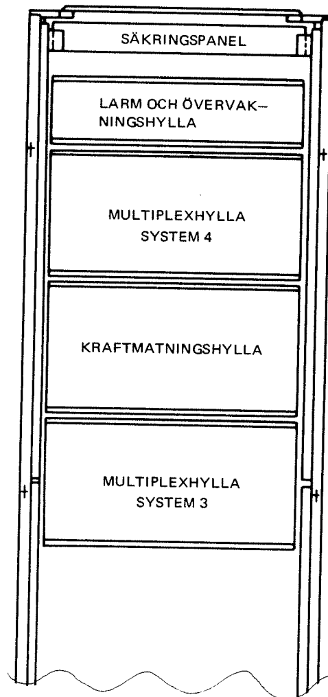
Bild 2. Terminalstation PCM
