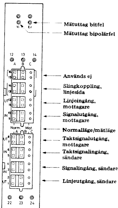
Bild 10. Kodomvandlarkortkrets bygglaceringar
