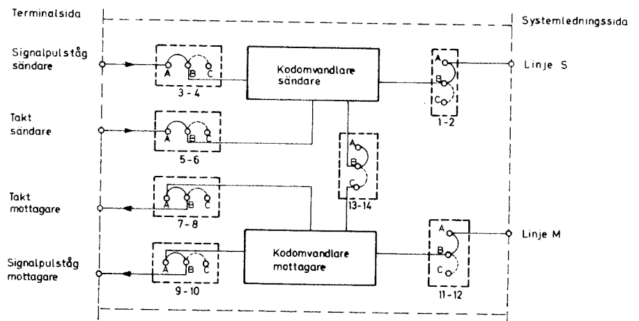
Bild 11. Blockschemata för omkopplingar på kodomvandlarkortet
