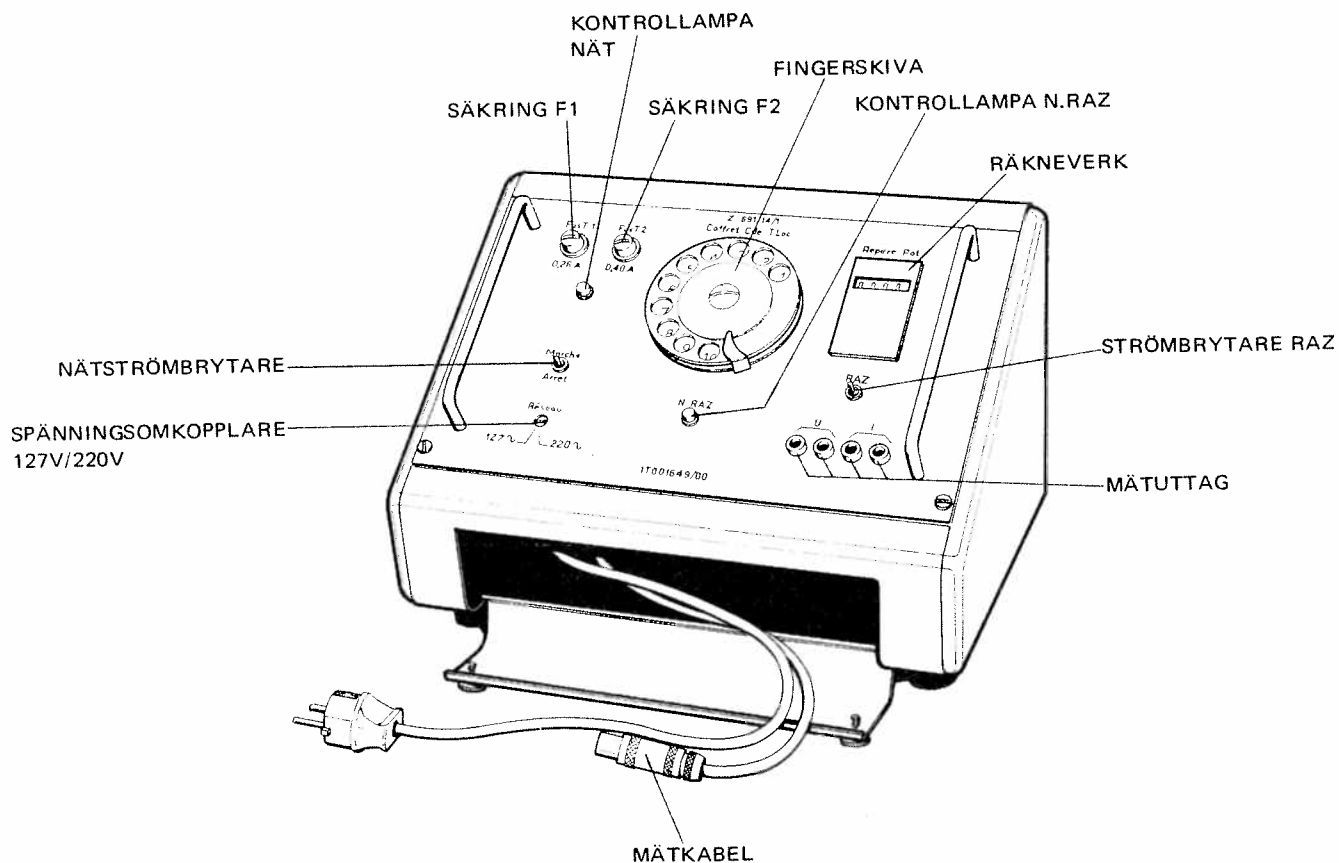
Bild 16. Lokalisering-instrument F5841-000021
