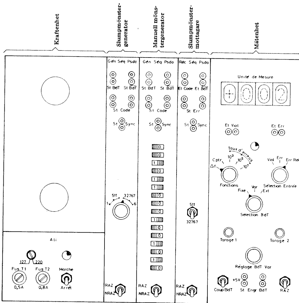
Bild 18. PCM-universalinstrument F5841-000001
