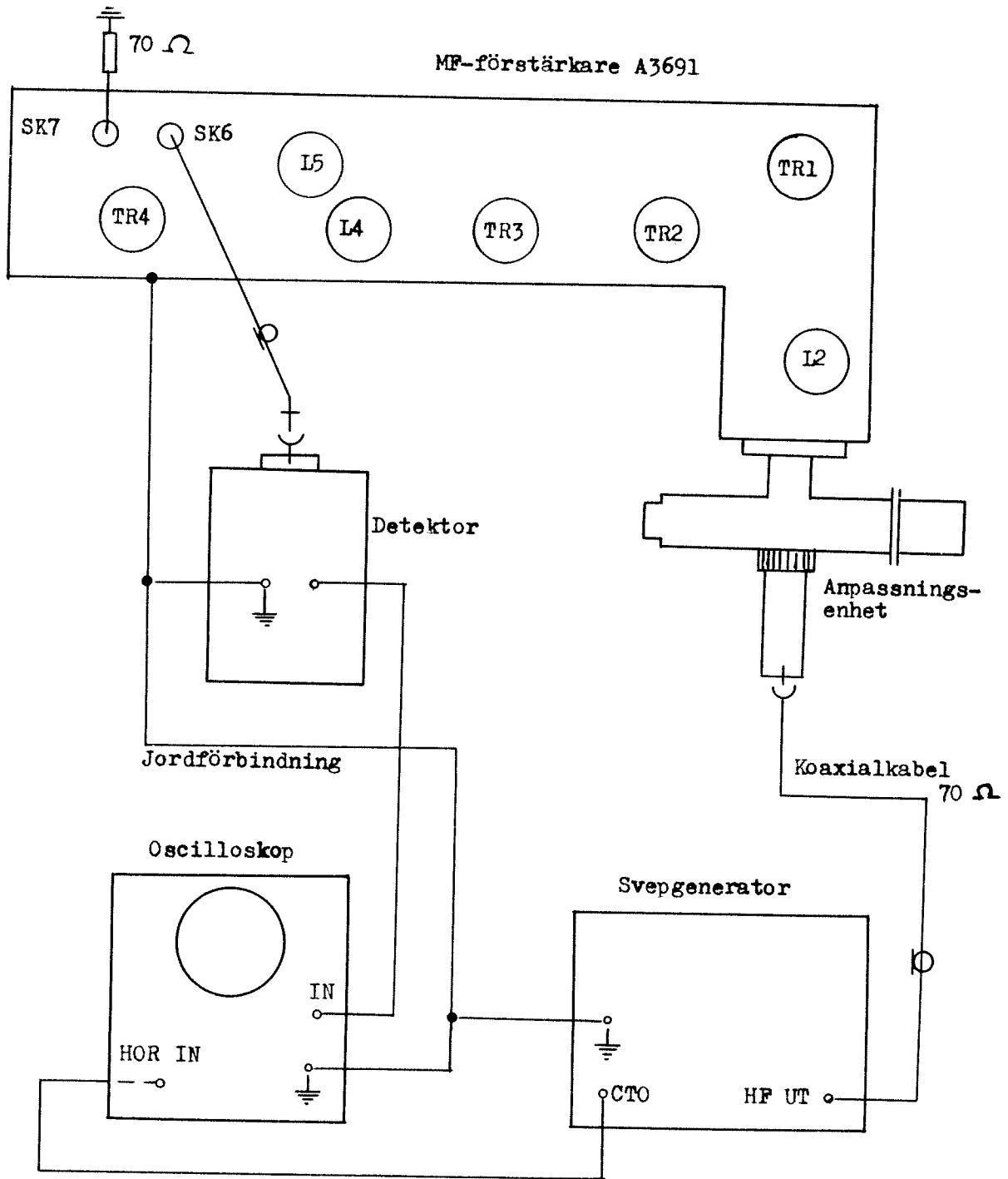
Bild 1. Uppkopplings-skiss, trimning MF-först. A 3691
