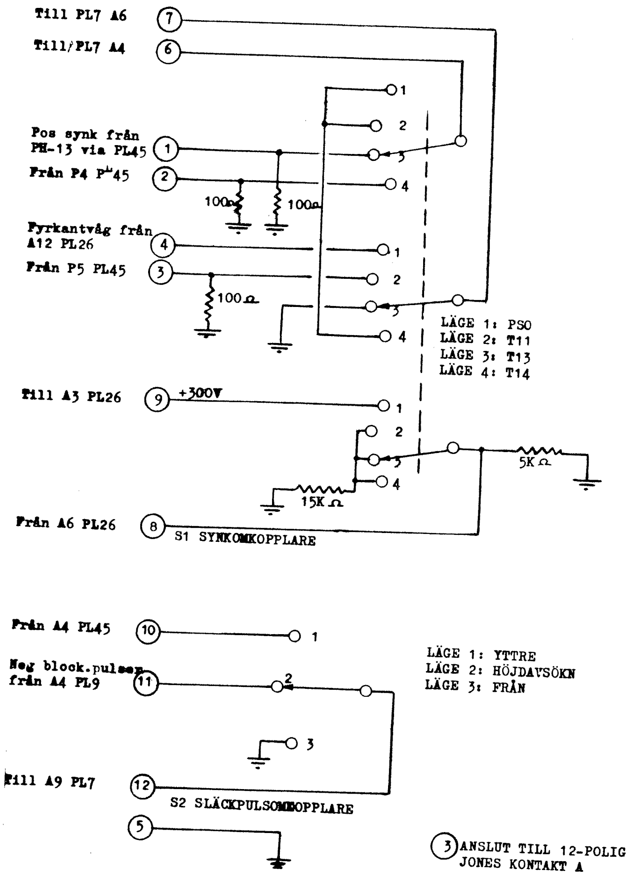
Bild 4. Principschema PL46.
