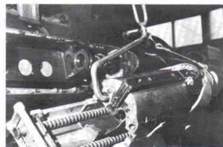
Bygeln vid lyft sedd snett bakifrån.
